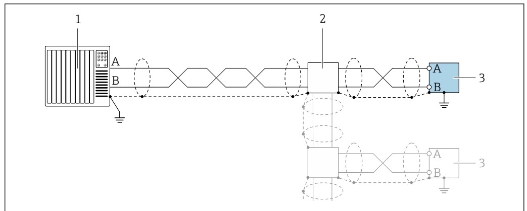
18 Пример подключения для Modbus RS485
