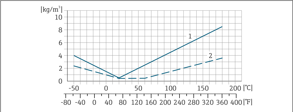
1 Калибровка по плотности на месте эксплуатации, в примере при +20 °C (+68 °F) 2 Расширенная калибровка плотности
