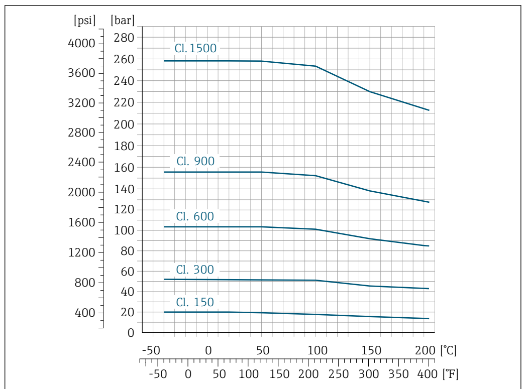
17 Avec matériau de bride inox, 1.4410/F53 25Cr Duplex (Super Duplex)
