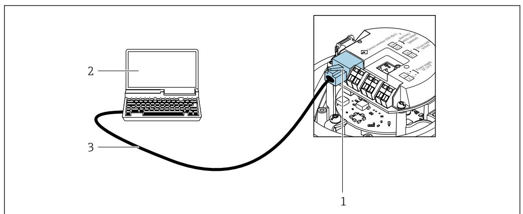
25 Raccordement pour caractéristique de commande "Sortie", Option B : 4-20 mA HART, sortie impulsion/fréquence/tor
