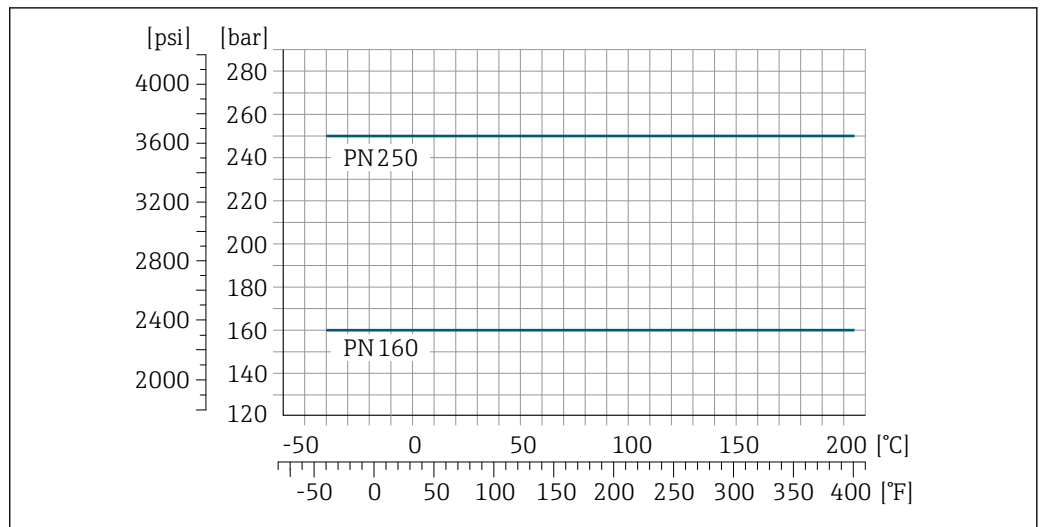
16 Avec matériau de bride inox, 1.4410/F53 25Cr Duplex (Super Duplex)
