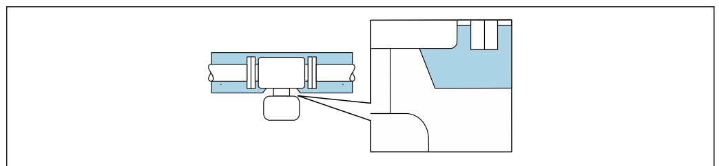
18 Isolation thermique avec tube prolongateur exposé
