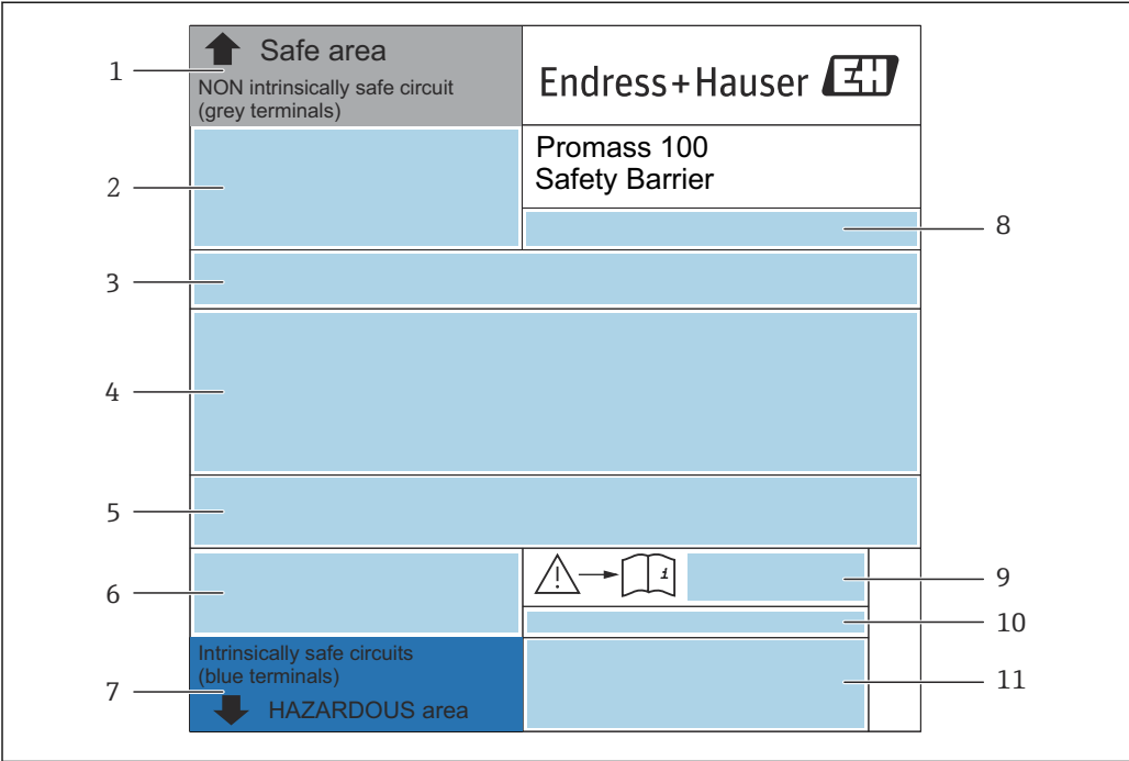
4 Пример заводской таблички искробезопасного барьера Promass 100 1 Невзрывоопасная зона или зона 2/разд. 2 2 Серийный номер, номер материала и двухмерный штрих-код искробезопасного барьера Promass 100 3 Данные электрического подключения, как доступные входы и выходы, сетевое напряжение 4 Информация о сертификации по оценке взрывозащиты 5 Предупреждение по технике безопасности 6 Информация в отношении связи 7 Искробезопасная зона 8 Место изготовления 9 Номер сопроводительного документа, имеющего отношение к технике безопасности 10 Разрешенная температура окружающей среды ( T_a ) 11 Маркировки CE, C-Tick
