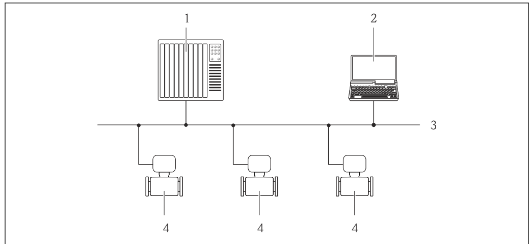
24 Opciones para la configuración a distancia mediante red PROFIBUS DP
