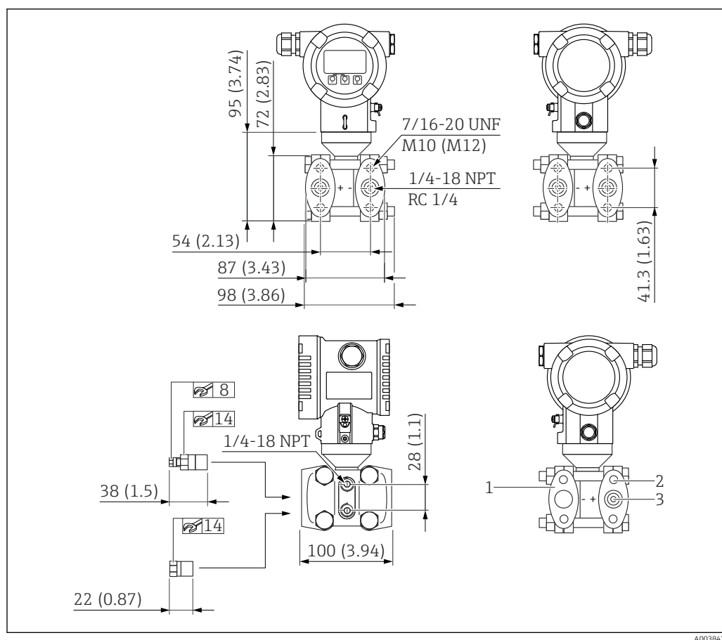
9 Вид спереди, вид слева-сбоку, вид справа-сбоку. Гайки всегда расположены на стороне низкого давления. Единица измерения мм (дюйм)
