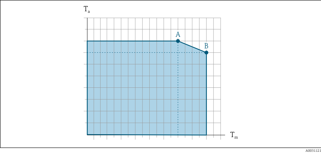
34 Representação exemplar, valores na tabela abaixo. T a Temperatura ambiente T m Temperatura do meio A Temperatura máxima permitida do meio T m a T a máx. = 60 °C (140 °F); temperaturas do meio mais altas T m requerem uma redução na temperatura ambiente T a B Temperatura ambiente T a máxima permitida para a temperatura média T m máxima especificada do sensor
