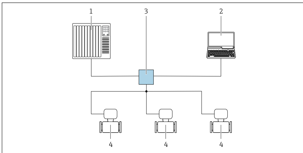
22 Opções para operação remota através da rede PROFIBUS: topologia estrela
