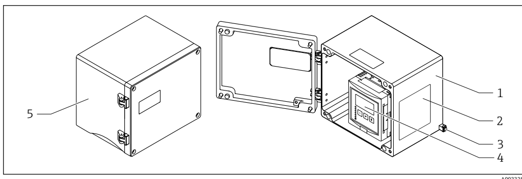
図 2 アルミニウム製フィールドハウジング内の Prosonic S の各部品
