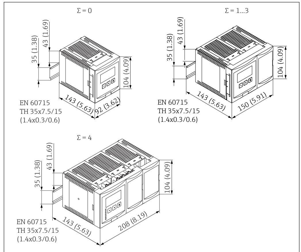
図 11 DIN レールハウジング付き Prosonic S の寸法 ; \Sigma : 追加の接続モジュール数。測定単位 mm (in)
