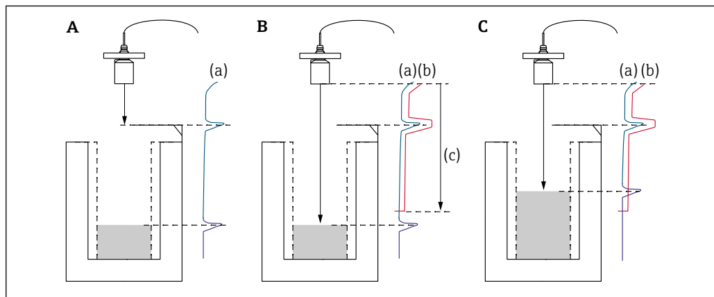
図 48 不要反射の抑制（マッピング）機能の動作原理
