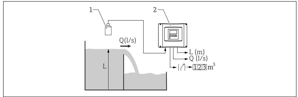
図 51 1つのセンサによるレベルと流量の同時測定
