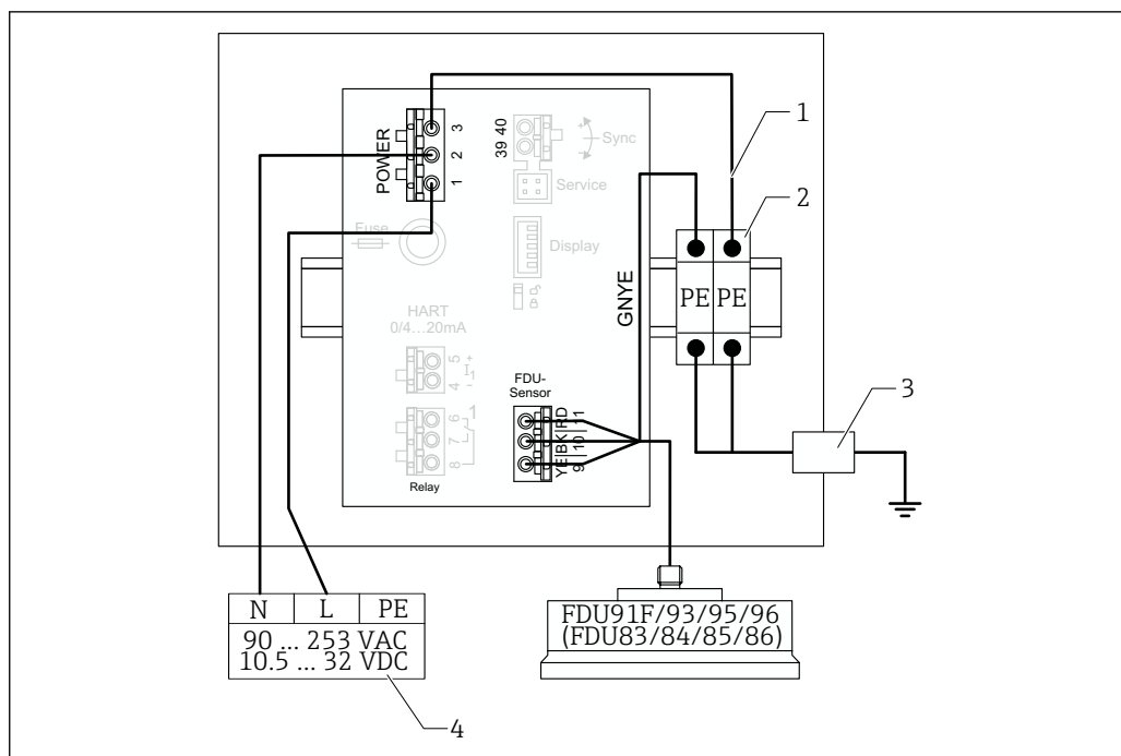
図 27 アルミニウム製フィールドハウジング内の金属製センサの電位平衡
