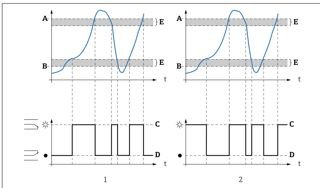
図 57 リミットタイプ = 「バンド内」または「バンド外」のパラメータ
