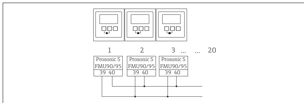
図 33 複数の FMU90/FMU95 変換器の同期
