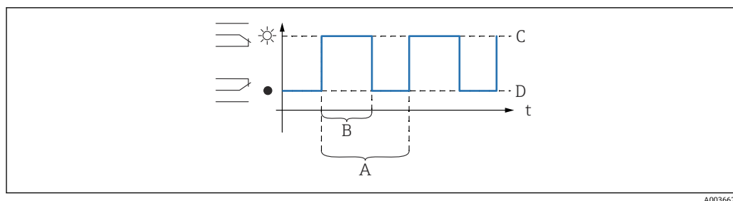
図 58 時間パルスリレーの設定
