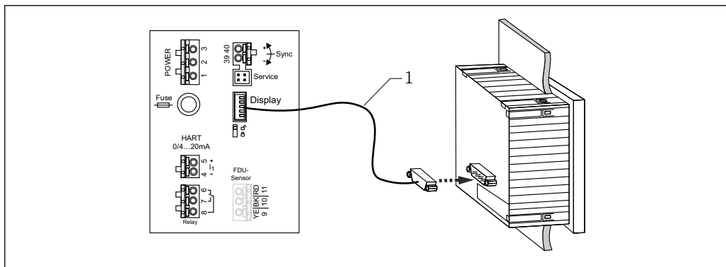
図 39 分離型ディスプレイと操作モジュールの接続
