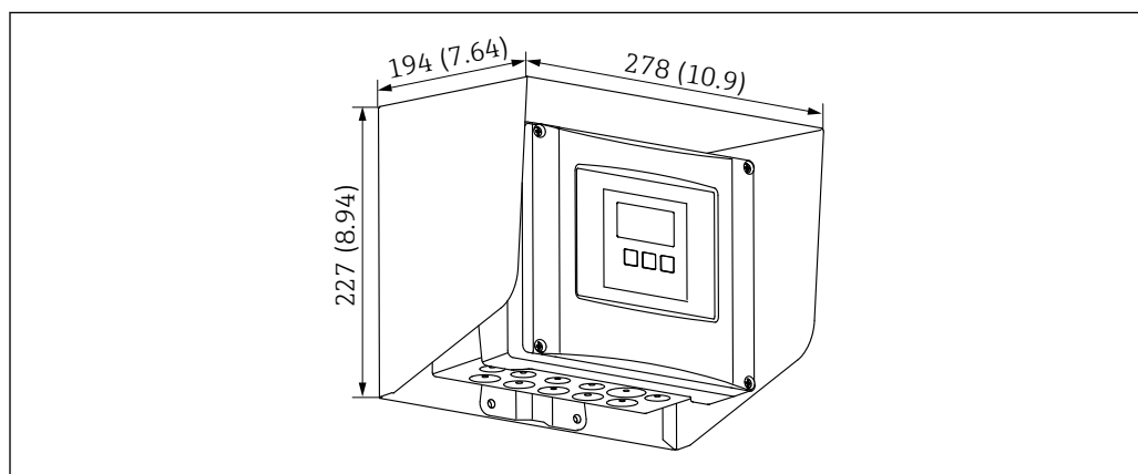
図 61 ポリカーボネート製フィールドハウジング用の日除けカバー。測定単位 mm (in)
