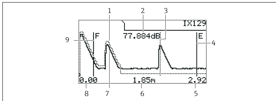
図 60 現場表示器での反射波形
