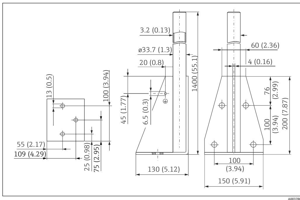
64 寸法。測定単位 mm (in)
