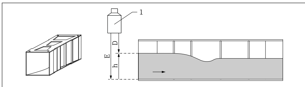
図 46 フリュームの空校正
