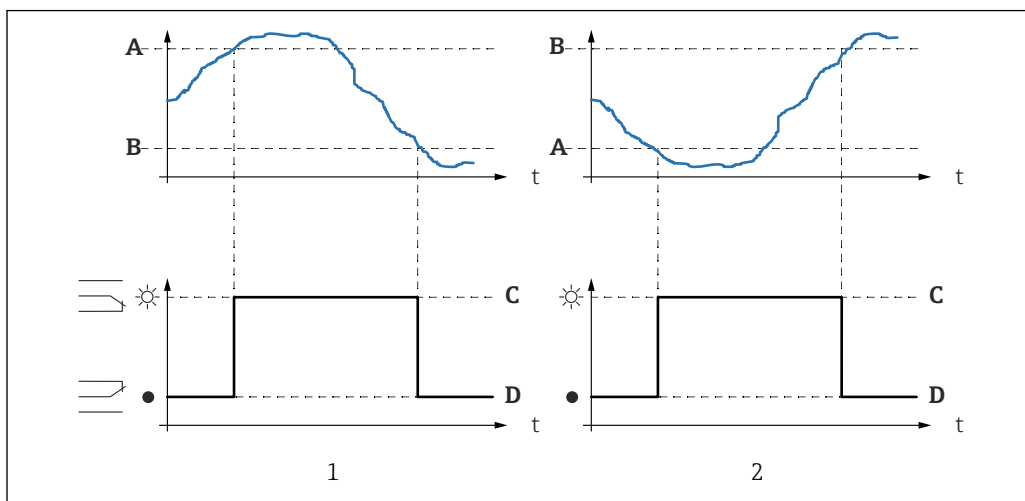
図 56 「リミットタイプ」 = 「標準」または「傾向/速度」のパラメータ
