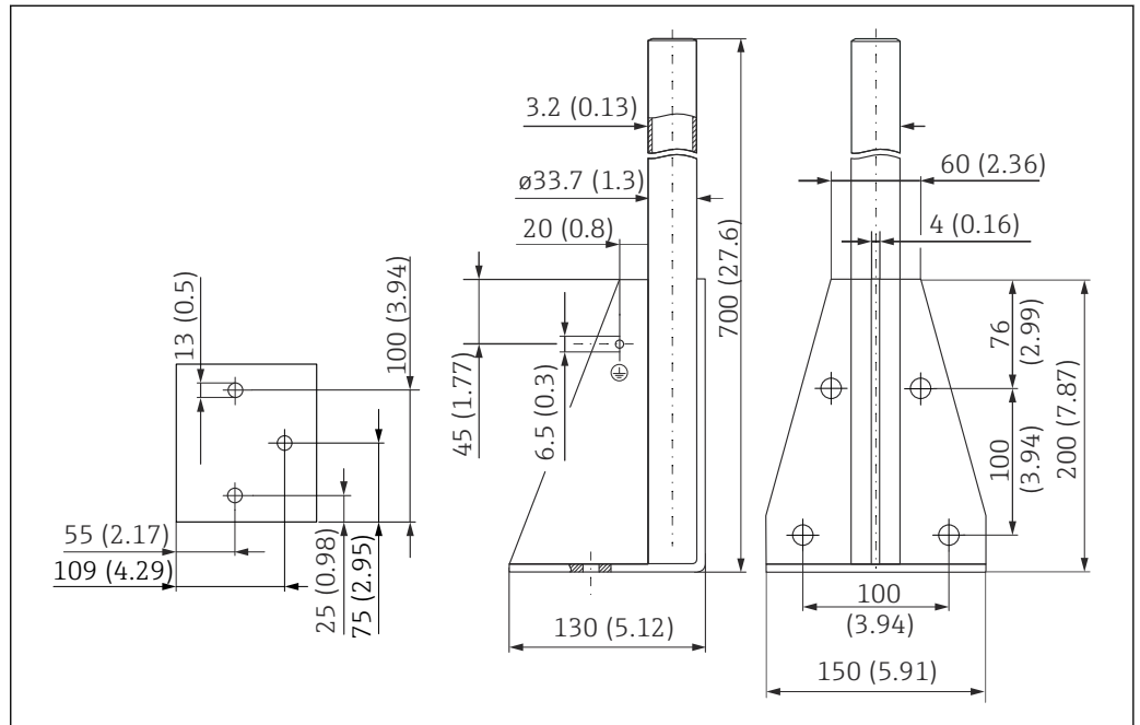
図 63 寸法。測定単位 mm (in)
