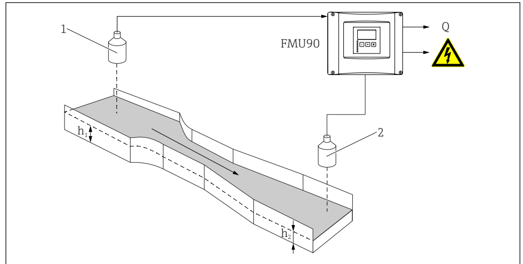
図 49 2つの超音波センサを使用したバックウォーターディテクション
