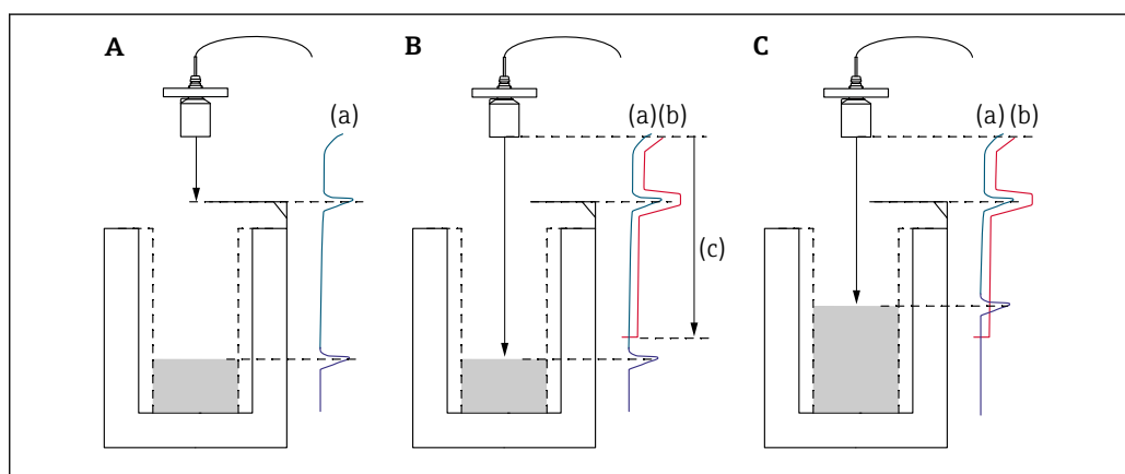
図 50 マッピング（不要反射の抑制）機能の動作原理
