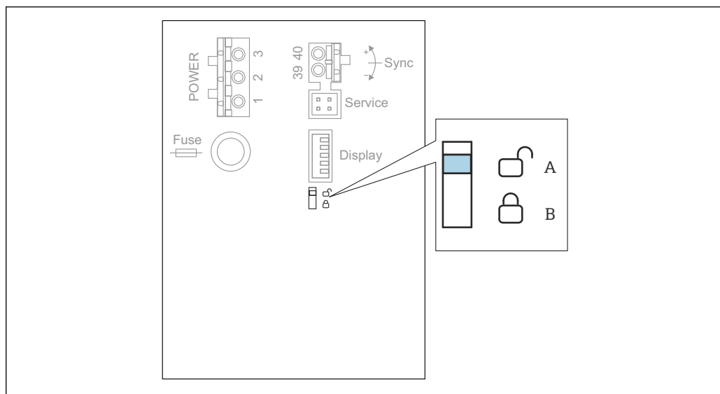
図 59 ハードウェアのロック
