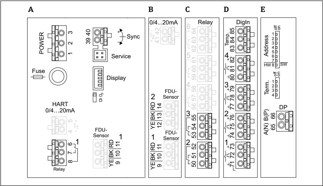
図 21 Prosonic S 用の端子 (一部の機器バージョンには、灰色で示された端子はありません。)
