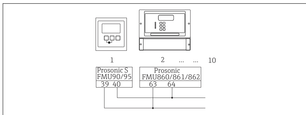
図 34 FMU90/FMU95 と FMU86x の同期
