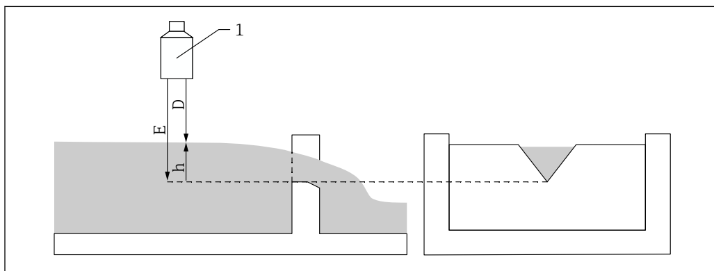
図 47 堰の空校正
