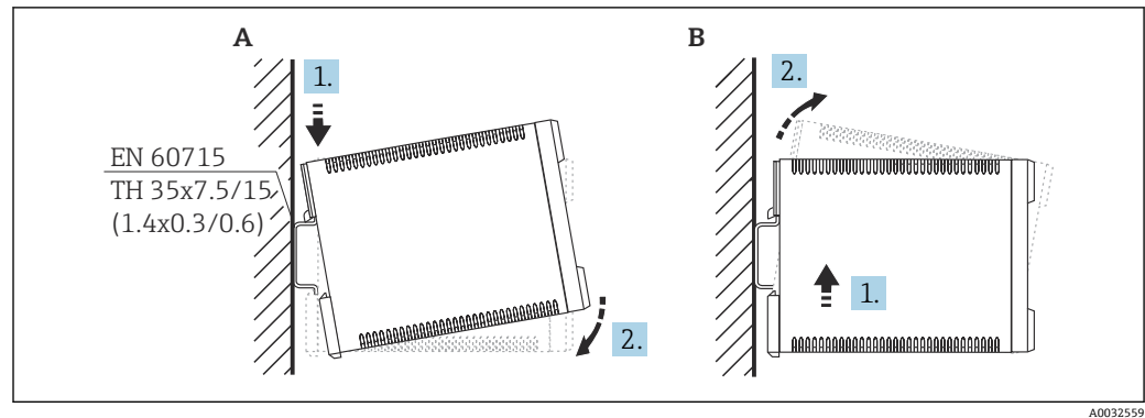
12 DIN レールハウジングの取付け/取外し。測定単位 mm (in)
