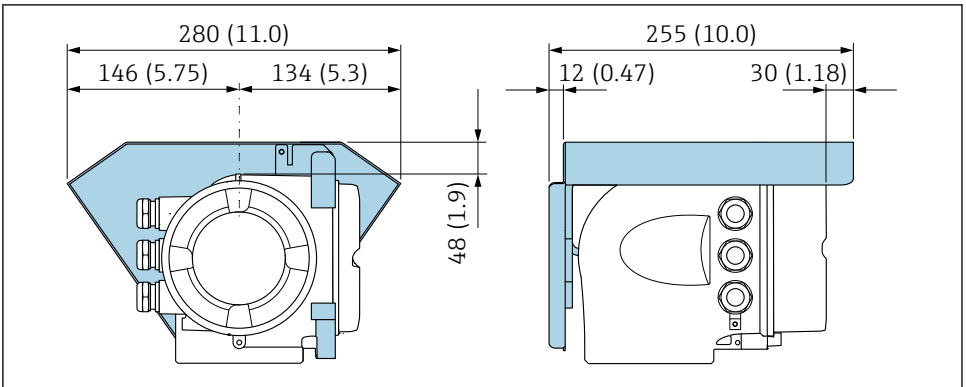
4 Tapa de protección ambiental para Proline 500; unidad mm (in)
