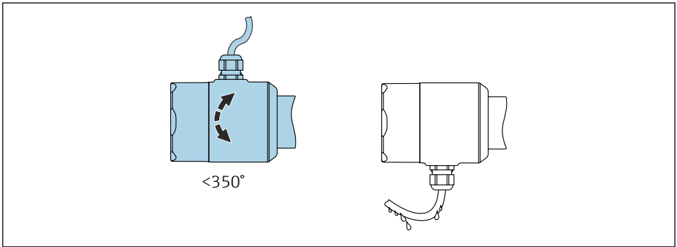
16 Custodia senza vite di bloccaggio esterna e con anello salvagoccia
