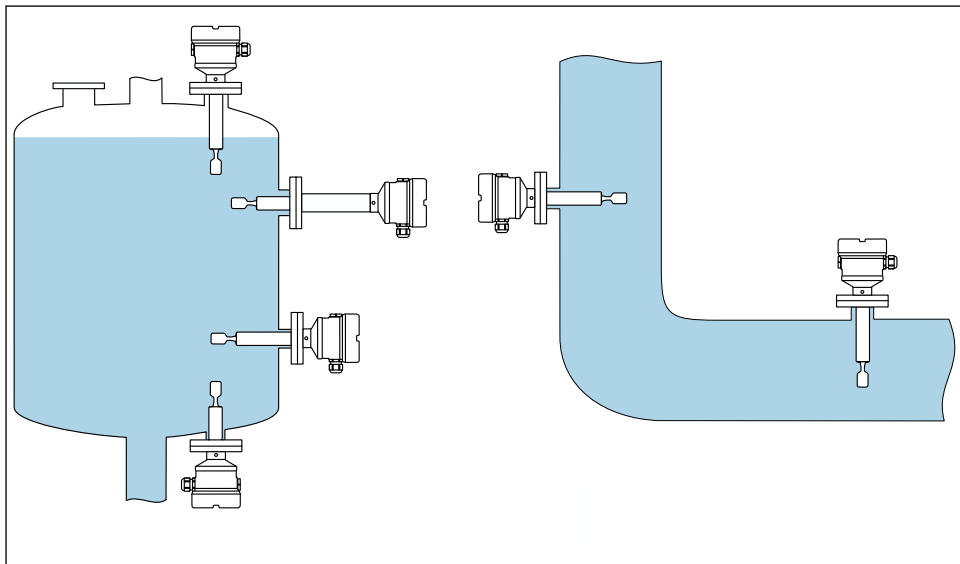
4 Esempi di installazione in recipiente, serbatoio o tubo
