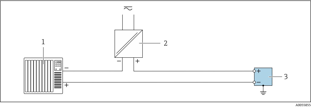
図 10 パルス出力/周波数出力/スイッチ出力（パッシブ）の接続例 1 オートメーションシステム、パルス入力/周波数入力/スイッチ入力付き（例：PLC） 2 電源 3 変換器、パルス出力/周波数出力/スイッチ出力（パッシブ）付き
