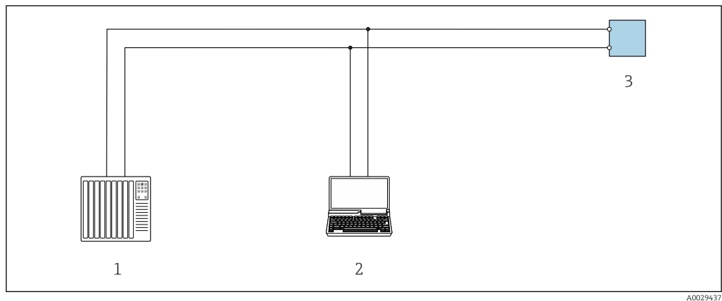
33 Options de configuration à distance via protocole Modbus RS485 (active)
