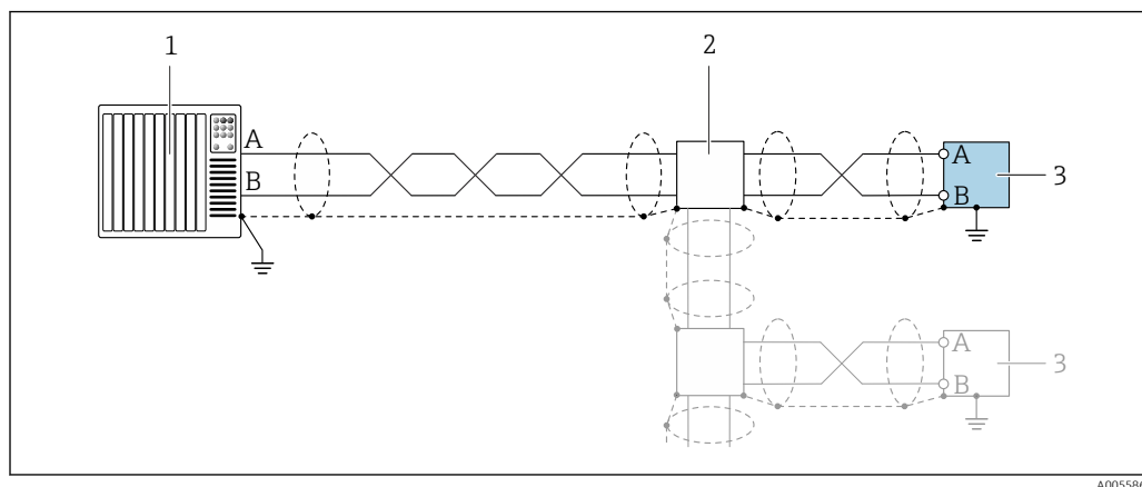
27 Exemple de raccordement pour Modbus RS485
