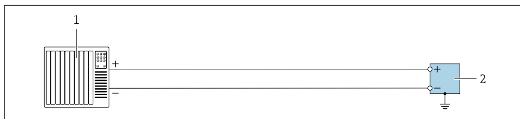
23 Exemple de raccordement pour sortie impulsion / sortie fréquence / sortie tout ou rien (active)
