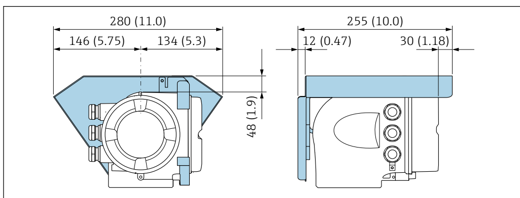
■ 12 Capot de protection climatique pour Proline 500 – unité mm (in)
