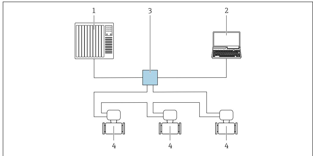
☒ 30 Options de configuration à distance via réseau PROFINET : topologie en anneau
