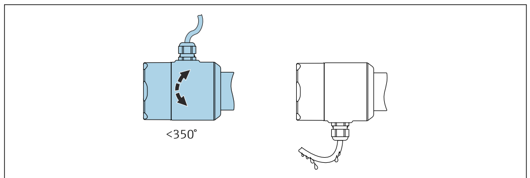
16 Invólucro sem parafuso de ajuste; forme um loop de gotejamento no cabo.
