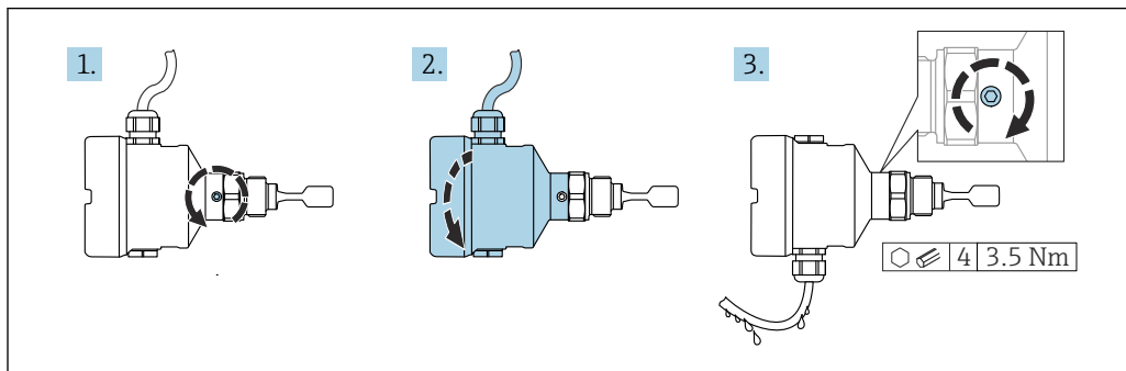
17 Invólucro com parafuso de bloqueio externo; forme um loop de gotejamento no cabo
