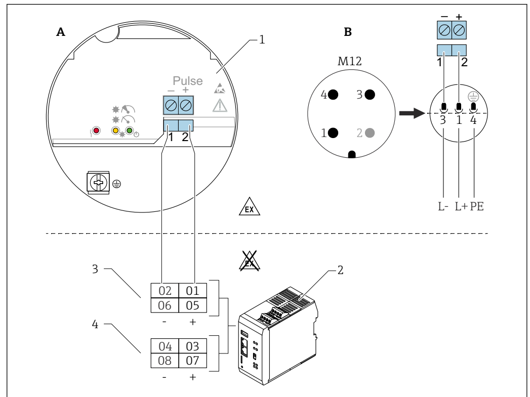
19 Diagrama de conexão: conexão da unidade eletrônica FEL60D com a calculadora de densidade QML51
