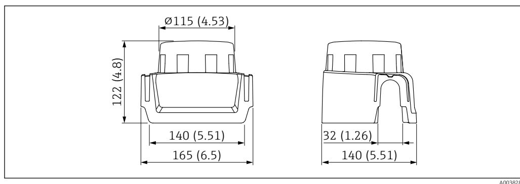
23 Tampa de proteção contra tempo para invólucro de alumínio de compartimento único. Unidade de medida mm (in)
