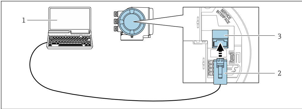
28 Conexão através de Interface de operação (CDI-RJ45)
