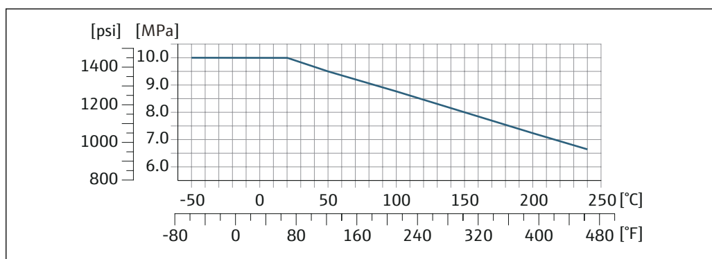
図 40 接続部の材質 1.4404 (SUS 316 または 316L 相当)
