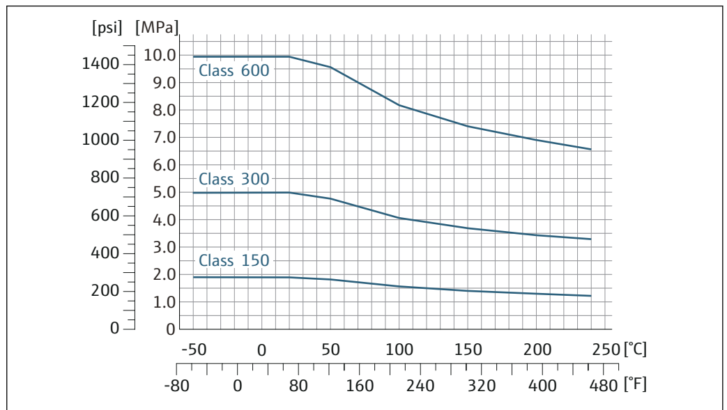
図 34 フランジ材質 1.4301 (SUS F304 相当) ; 接液部 アロイ C22
