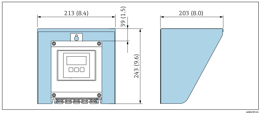
図 44 Proline 500 - デジタル用の日除けカバー
