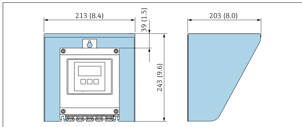
図 50 Proline 500 - デジタル用の日除けカバー
