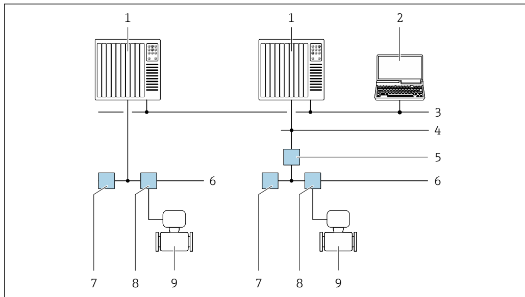
図 60 FOUNDATION フィールドバスネットワークを介したリモート操作のオプション
