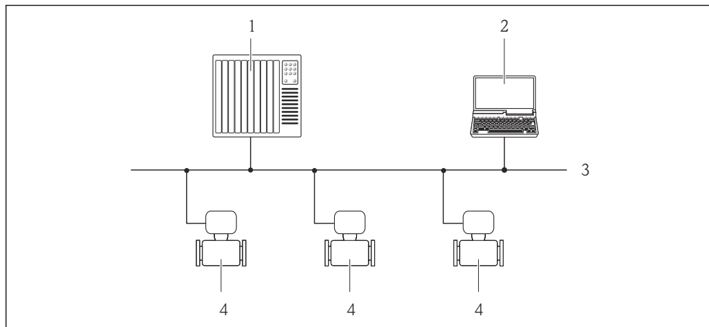
図 61 PROFIBUS DP ネットワークを介したリモート操作のオプション
