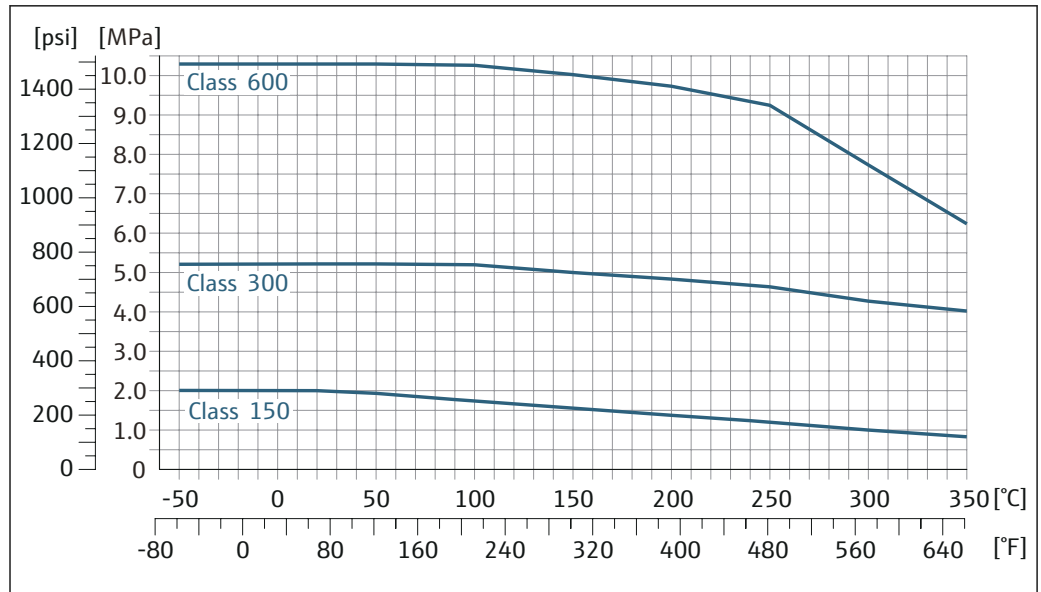
図 30 フランジ材質 アロイ C22
