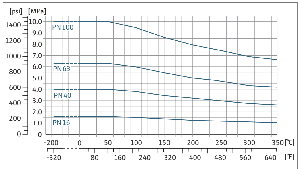
図 28 フランジ材質 1.4404 (SUS F316 または F316L 相当)、アロイ C22
