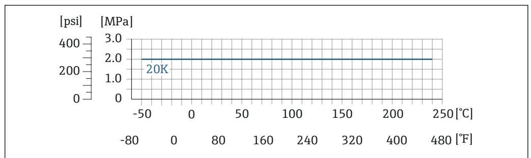
図 35 フランジ材質 1.4301 (SUS F304 相当) ; 接液部 アロイ C22
