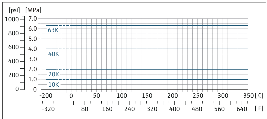
図 31 フランジ材質 1.4404 (SUS F316 または F316L 相当)、アロイ C22
