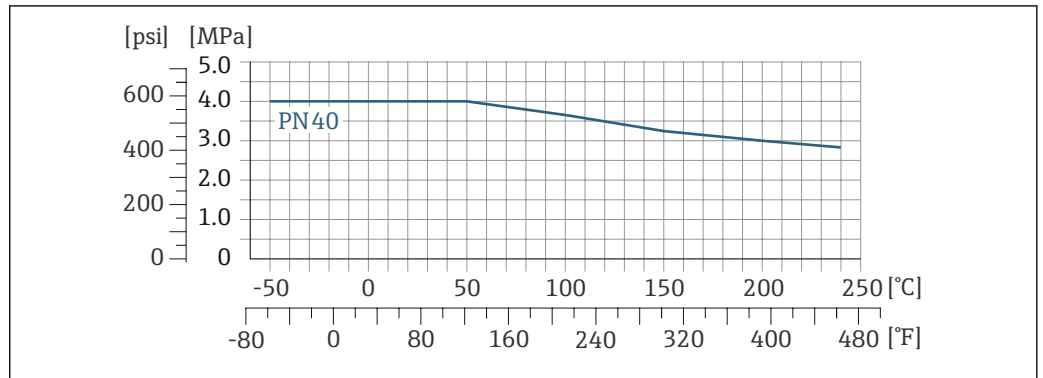
図 33 フランジ材質 1.4301 (SUS F304 相当) ; 接液部 アロイ C22
