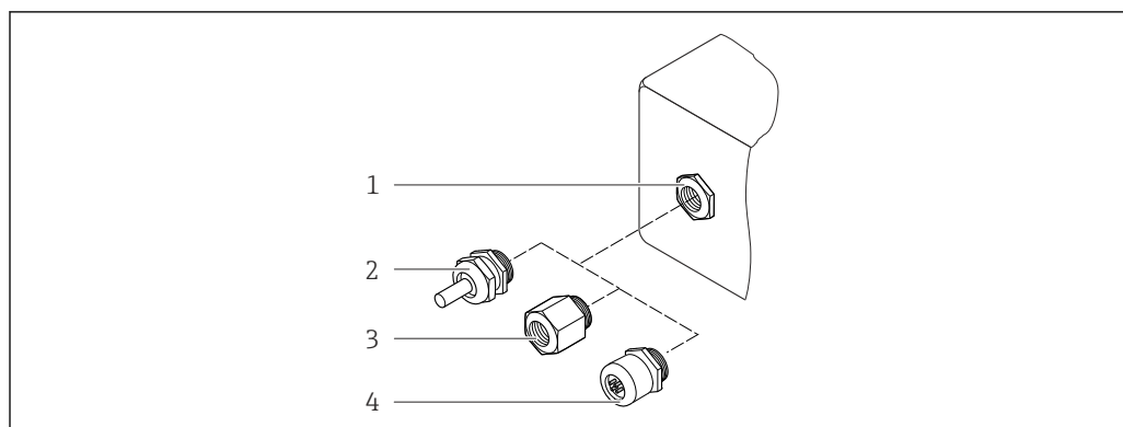
図 56 可能な電線管接続口/ケーブルグランド
