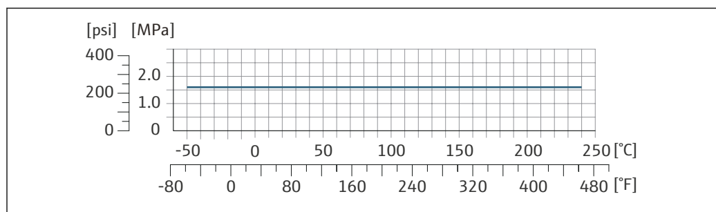
図 38 接続部の材質 1.4404 (SUS 316 または 316L 相当)
