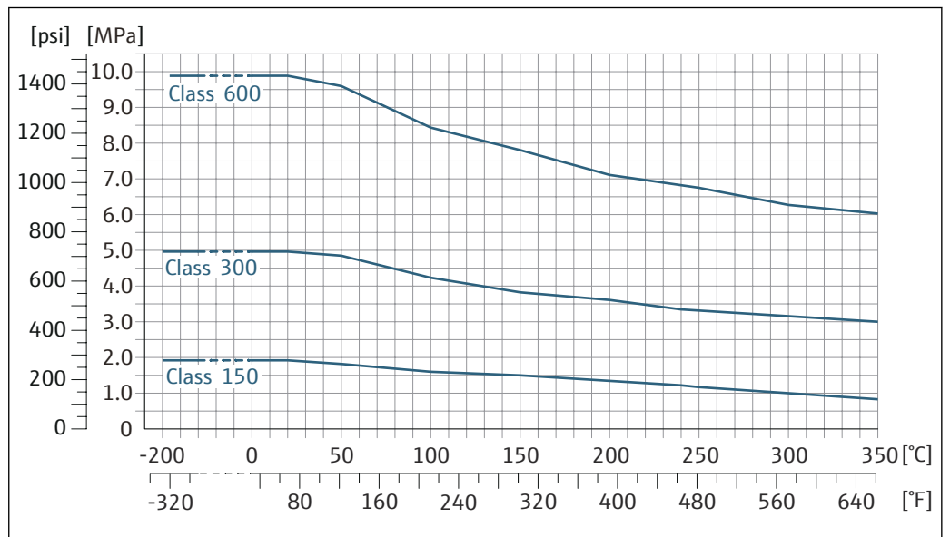
図 29 フランジ材質 1.4404 (SUS F316 または F316L 相当)
