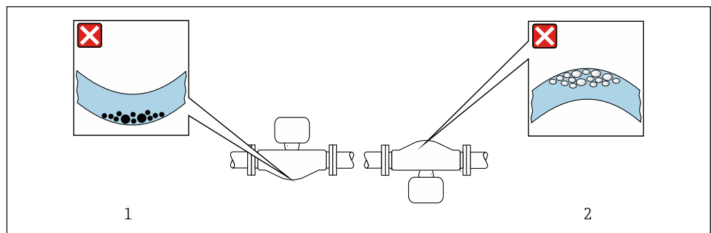
22 弓形計測チューブセンサの取付方向
