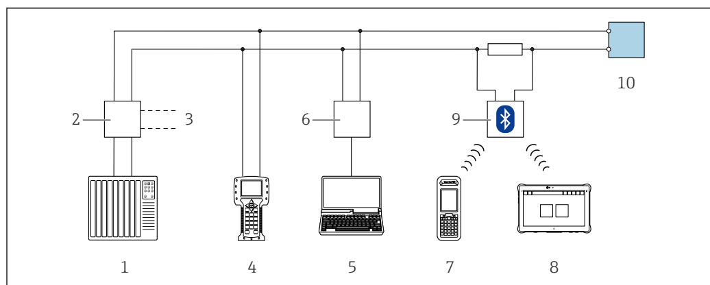
図 59 HART プロトコル経由のリモート操作オプション (パッシブ)
