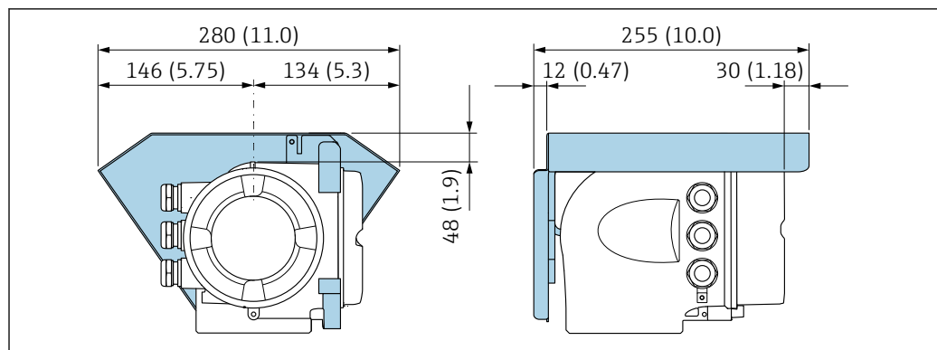
図 51 Proline 500 用の日除けカバー
