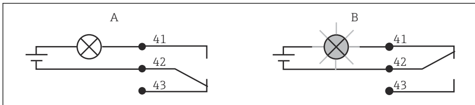
14 Commutazione di sicurezza consigliata per il contatto di allarme
