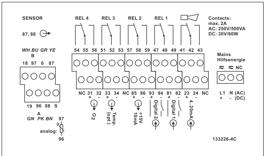
11 Etichetta del vano connessioni Liquisys M, versione WX/WS
