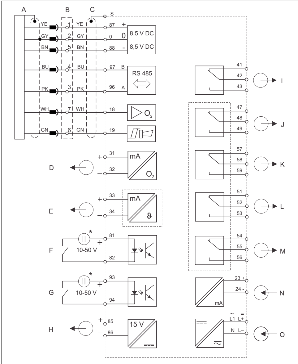
10 Collegamento elettrico del Liquisys M COM223/253 nella versione WX o WS
