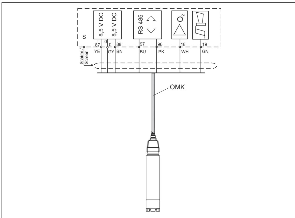
13 Esempio di connessione: COS31/71 con cavo OMK
