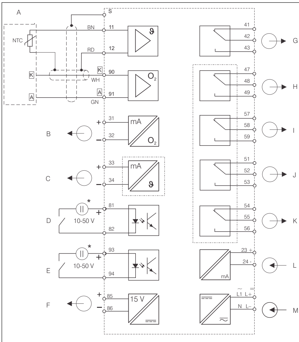
7 Collegamento elettrico del trasmettitore, versione DX o DS
