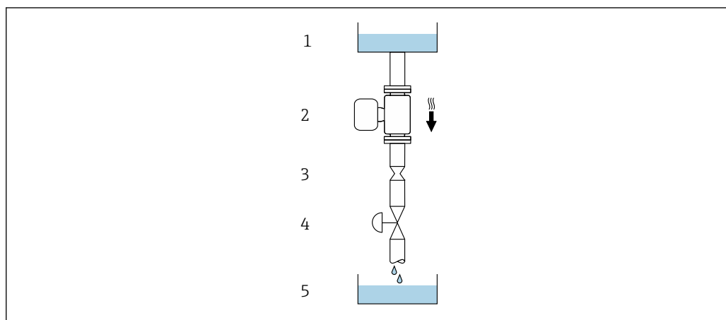
7 Montage dans un écoulement gravitaire (p. ex. applications de dosage)
