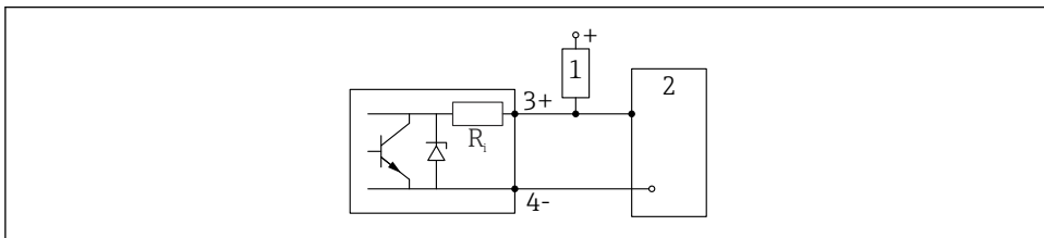
图 9 数字量输入的连接示例
