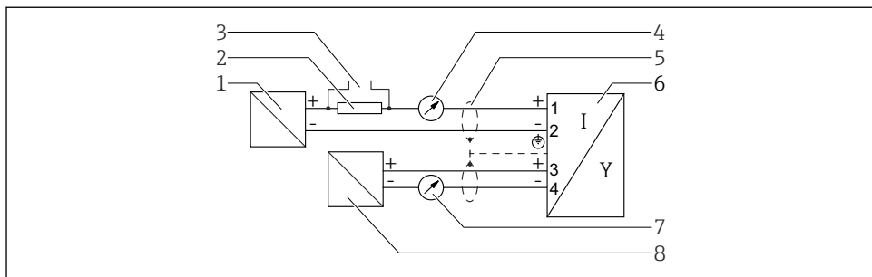
10 功能框图: 4 ... 20 mA HART + 4 ... 20 mA 模拟量
