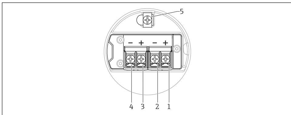
图 13 接线腔中的接线端子分配; 4 ... 20 mA HART + 4 ... 20 mA 模拟量; 双腔室外壳
