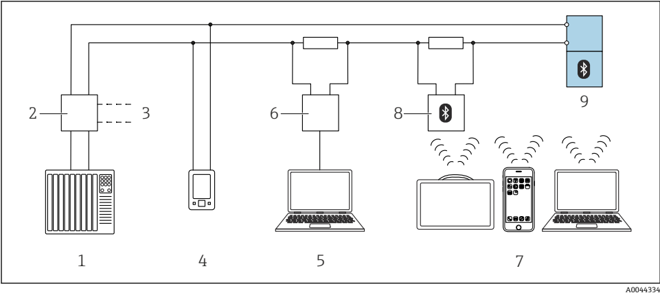
图 21 通过 HART 通信实现远程操作
