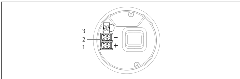
图 11 接线腔内的接线端子和接地端，单腔室外壳
