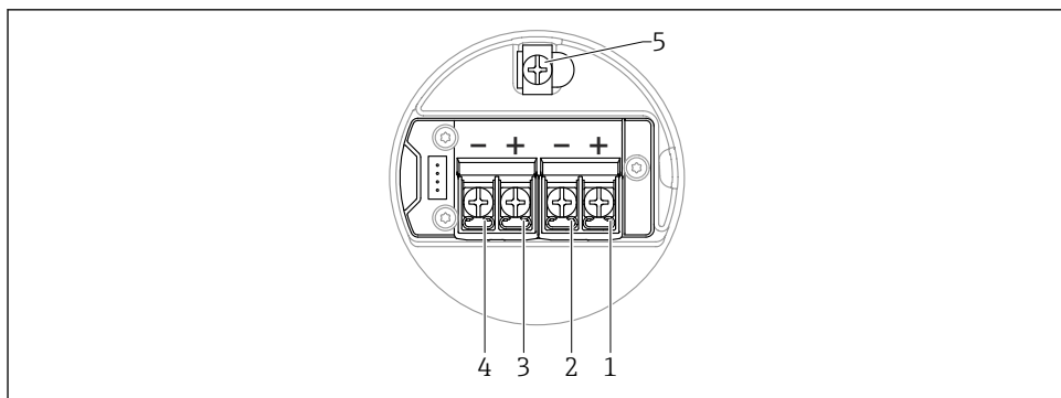
图 17 接线腔中的接线端子分配; 4 ... 20 mA HART, 开关量输出; 双腔室外壳 (L 型)
