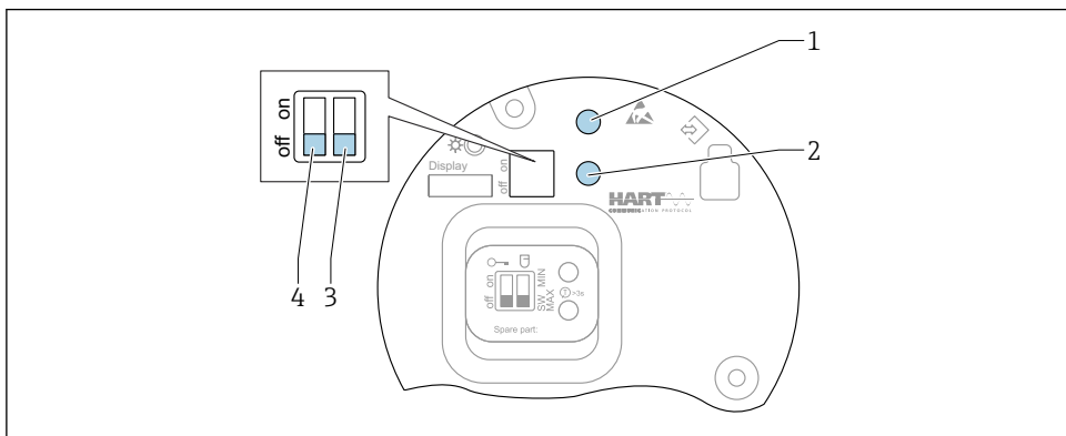
图 18 HART 电子插件上的操作按键和 DIP 开关
