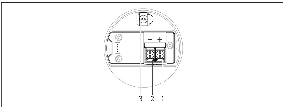
图 15 接线腔中的接线端子分配；4 ... 20 mA HART；双腔室外壳（L 型）
