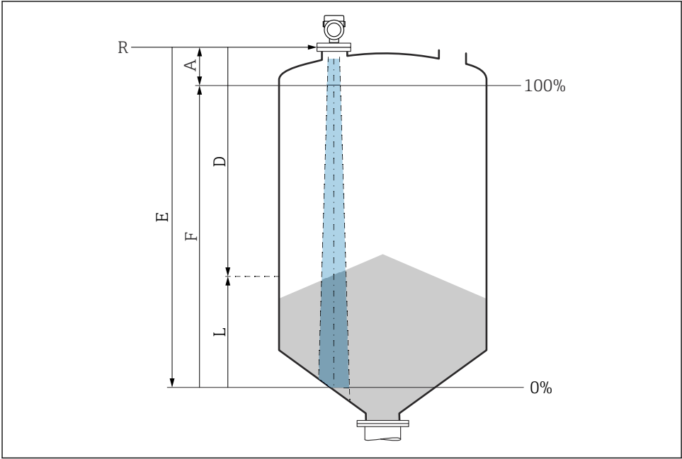
图 22 固体散料料位测量的设置参数
