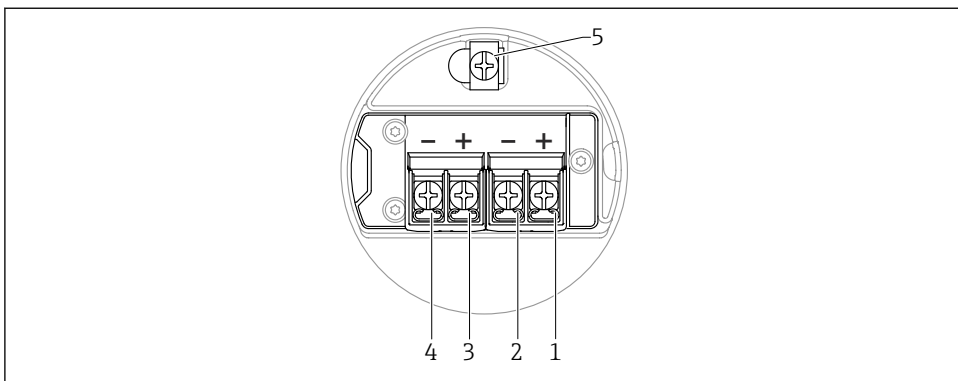
图 14 接线腔中的接线端子分配；4 ... 20 mA HART，开关量输出，双腔室外壳
