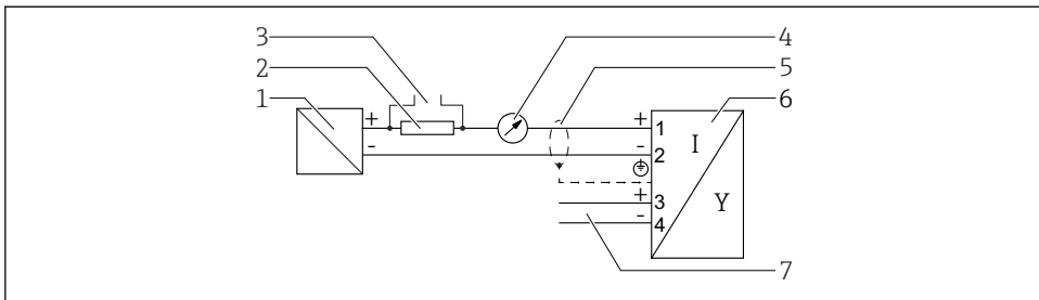
图 7 功能框图: 4 ... 20 mA HART, 开关量输出
