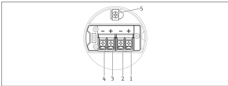
图 16 接线腔中的接线端子分配; 4 ... 20 mA HART + 4 ... 20 mA 模拟量; 双腔室外壳 (L 型)
