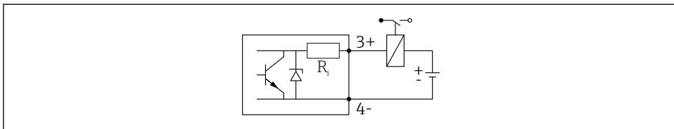
图 8 继电器的连接示例
