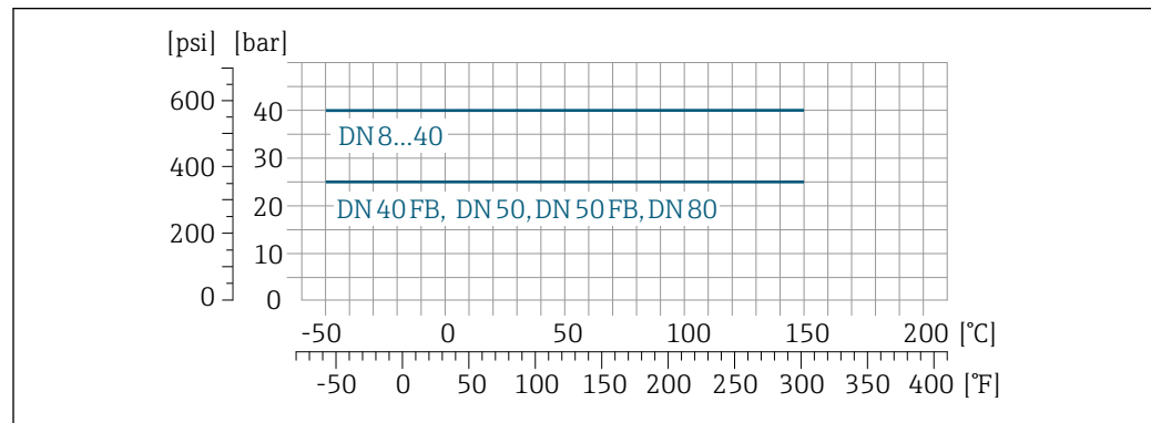
21 Avec matériau de raccord titane grade 2
