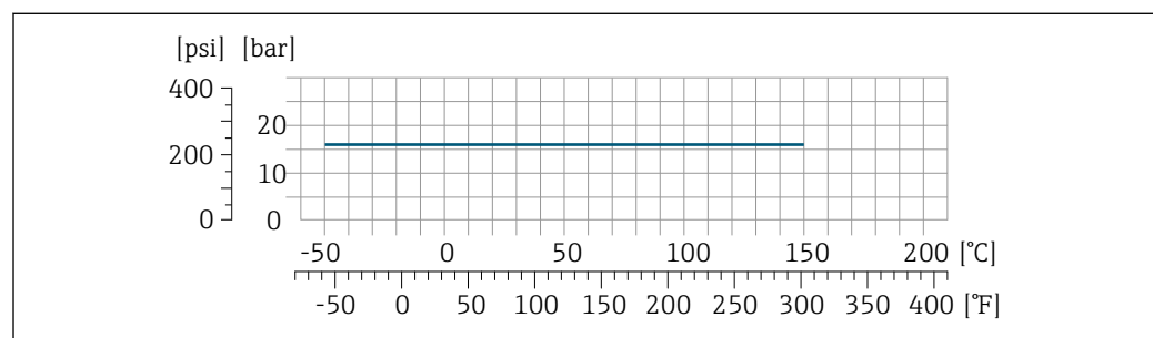
23 Avec matériau de raccord titane grade 2
