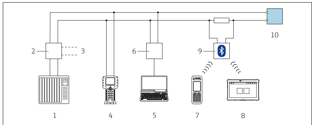
38 Options de configuration à distance via protocole HART (passive)
