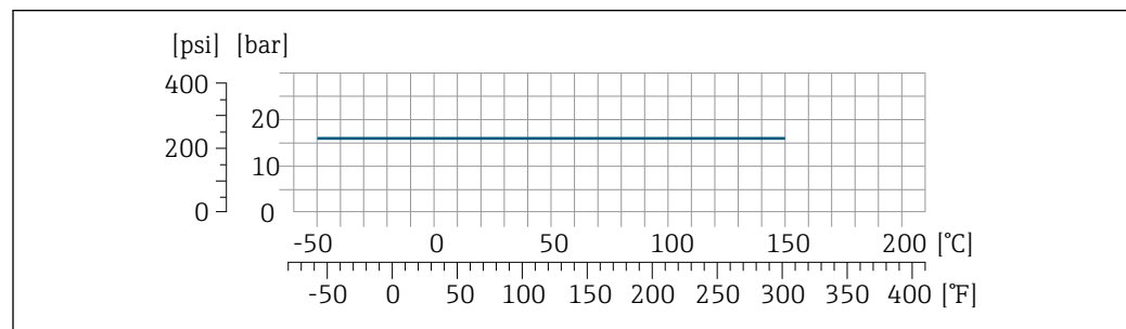
22 Avec matériau de raccord titane grade 2
