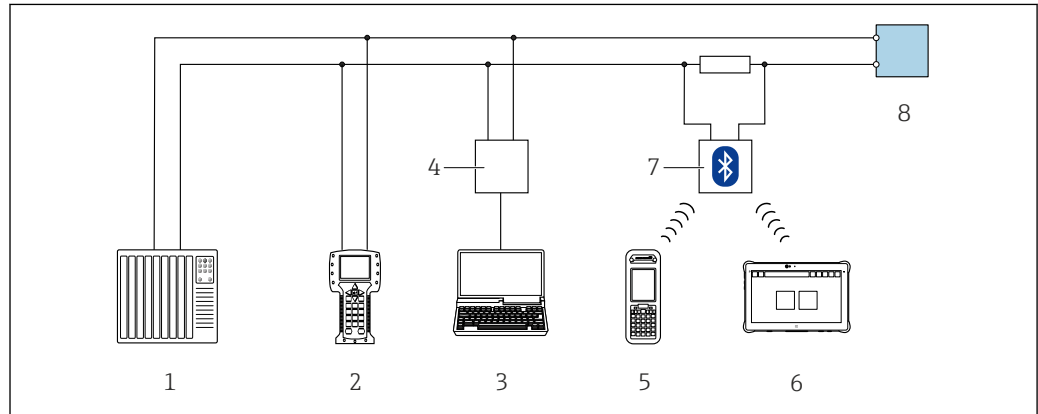
37 Options de configuration à distance via protocole HART (active)
