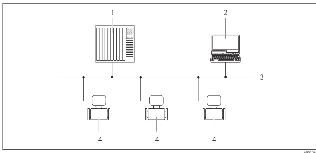
19 Варианты дистанционного управления через сеть PROFIBUS DP
