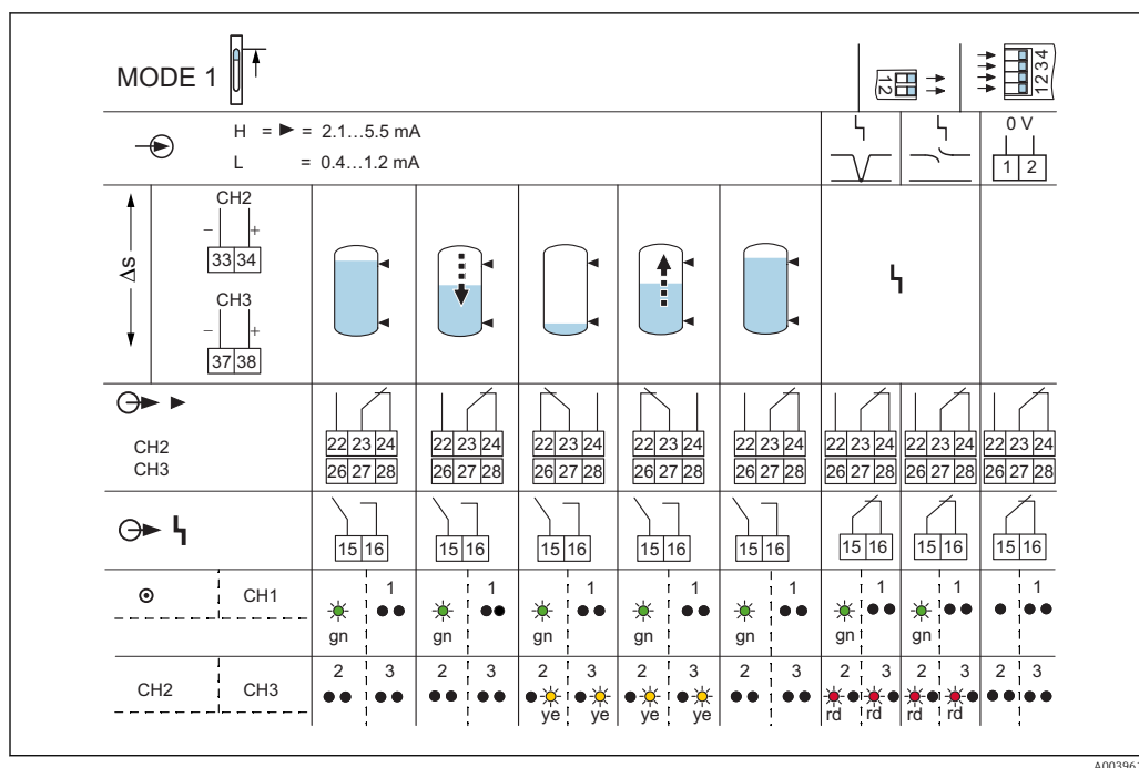
29 Comportamento de comutação e sinalização com erro de corrente H > 2.1 \text{ mA} (FEL56)
