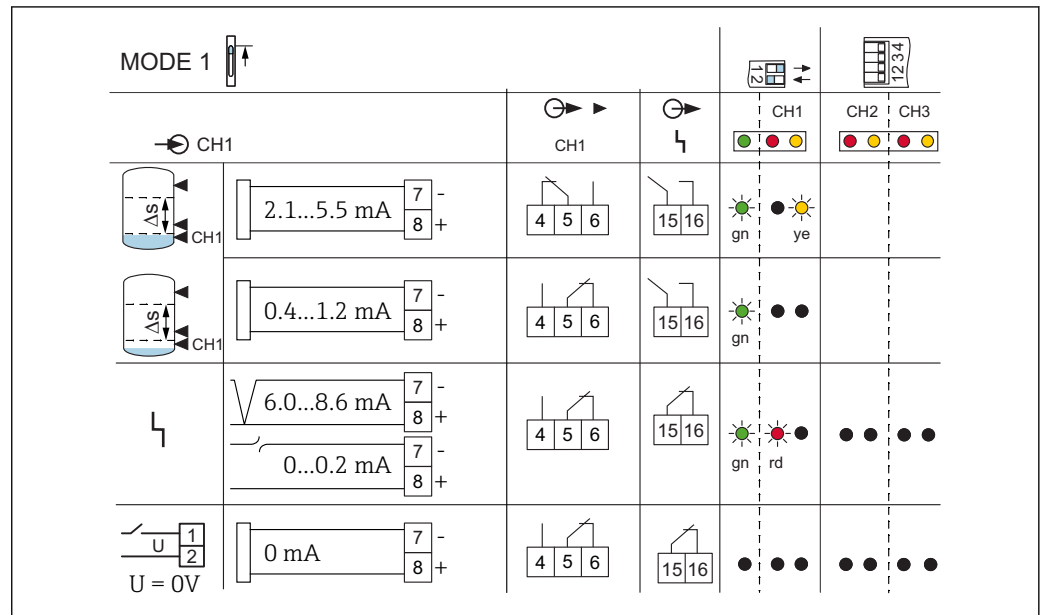
35 Comportamento de comutação e sinalização com erro de corrente L < 1.2 \text{ mA} (FEL48, FEL58, FEL68, FEM58, FEI58)
