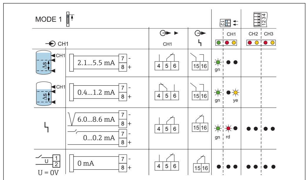
33 Comportamento de comutação e sinalização com erro de corrente H > 2.1 \text{ mA} (FEL56)
