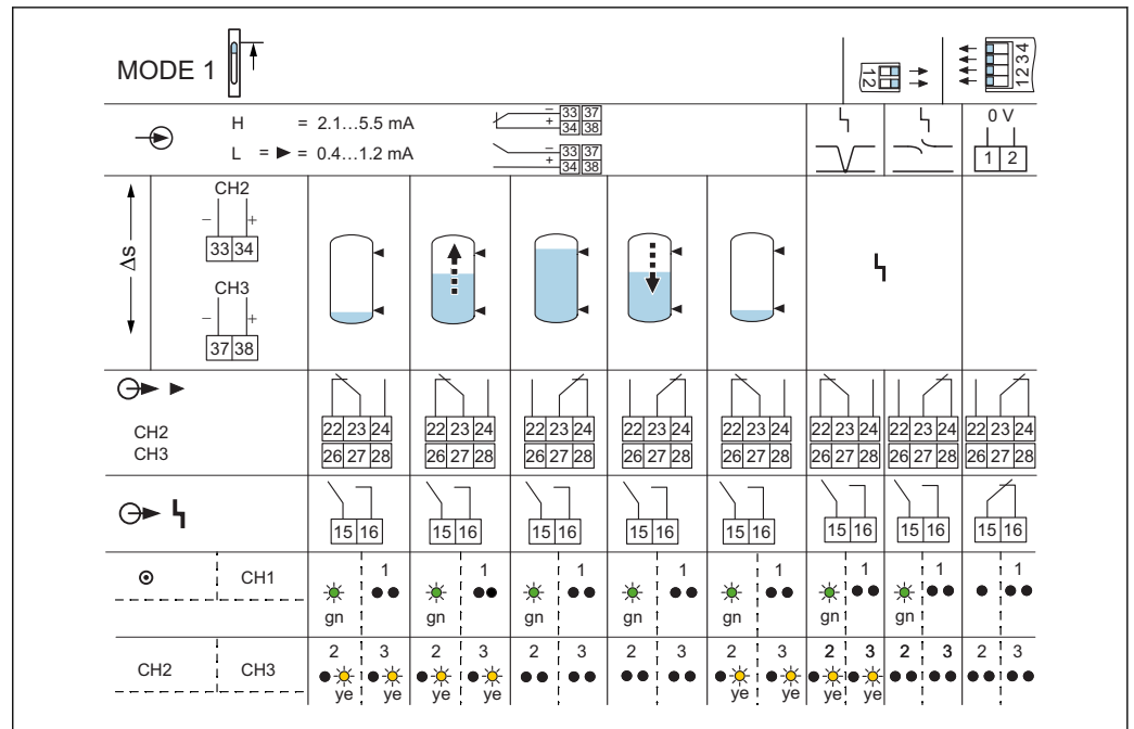
32 Comportamento de comutação e sinalização com corrente de erro L < 1.2 mA (FEL48, FEL58, FEL68, FEM58, FEI58)
