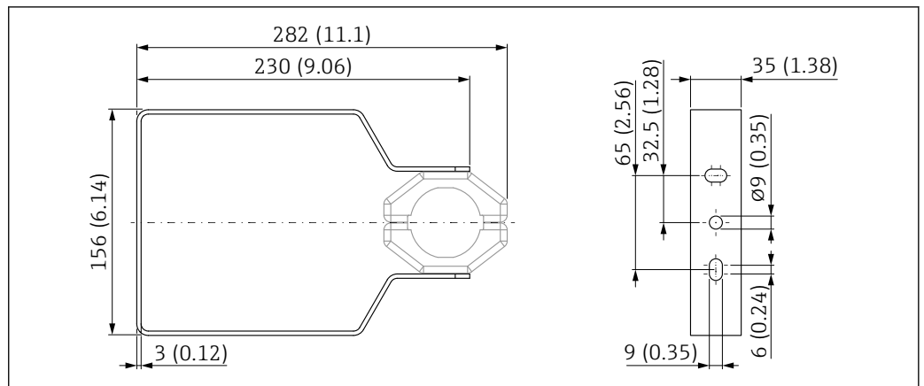
42 寸法；調整可能な取付ブラケット FMR6xB。測定単位 mm (in)
