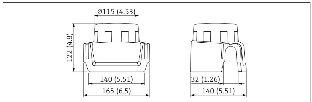
図 40 日除けカバー、プラスチック、XW111 の寸法。測定単位 mm (in)
