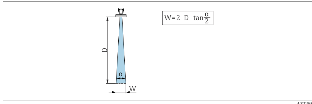
図 8 ビーム放射角 \alpha 、距離 D 、ビーム幅 W の関係
