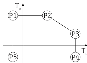
図 11 プラスチックハウジング ; プロセス温度 -40 \sim +130 \text{ }^{\circ}\text{C} ( -40 \sim +266 \text{ }^{\circ}\text{F} )
