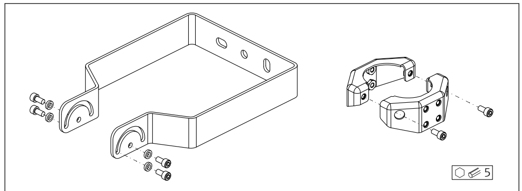
43 納入範囲；調整可能な取付ブラケット FMR6xB
