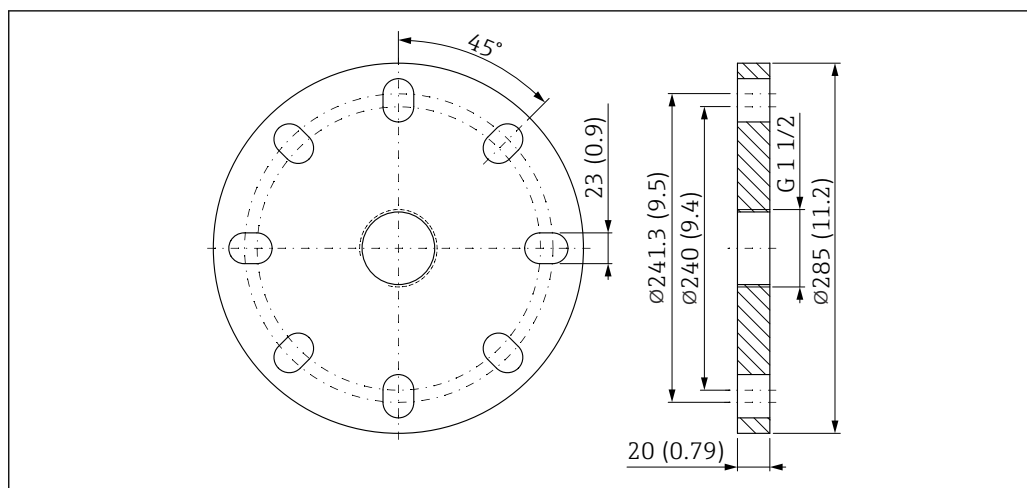
図 34 UNI フランジ 6"/DN150/150A の寸法。測定単位 mm (in)
