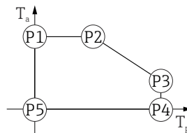
図 10 プラスチックハウジング ; プロセス温度 0 \sim +80 \text{ }^{\circ}\text{C} ( +32 \sim +176 \text{ }^{\circ}\text{F} )、CSA C/US 認定取得
