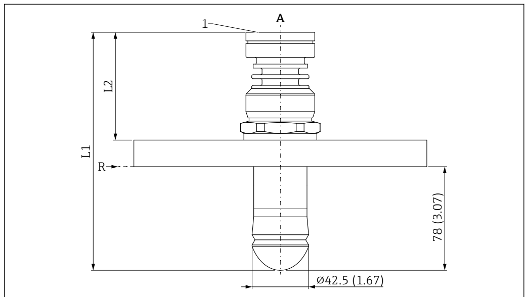
図 31 ドリップオフアンテナ 50 mm (2 in) (UNI フランジプロセス接続) の寸法。測定単位 mm (in)
