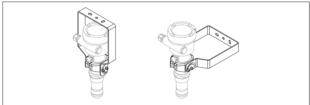
図 41 調整可能な取付ブラケット FMR6xB；天井または壁面取付け
