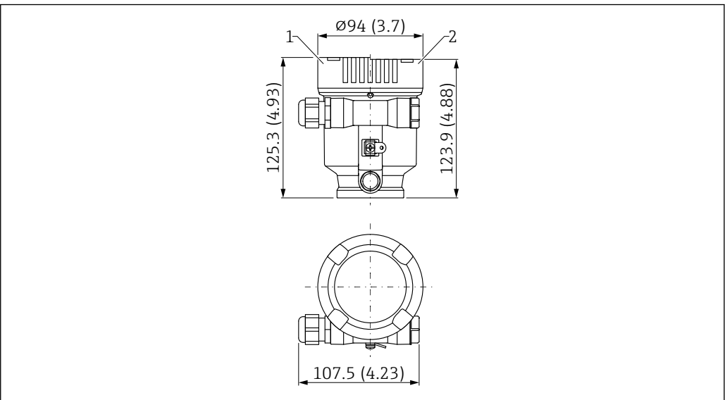
図 19 寸法；シングルコンパートメントハウジング（プラスチック）；M20 カップリングおよびプラグ（プラスチック）付き。測定単位 mm (in)
