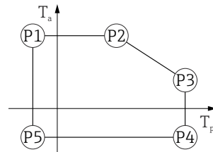
図 13 アルミニウムハウジング ; コーティング ; プロセス温度 -40～+80 °C (-40～+176 °F)
