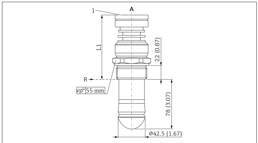
図 30 ドリップオフアンテナ 50 mm (2 in)、ネジ込みプロセス接続の寸法
