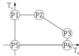
図 12 プラスチックハウジング ; プロセス温度 0～+130 °C (+32～+266 °F)、CSA C/US 認定取得
