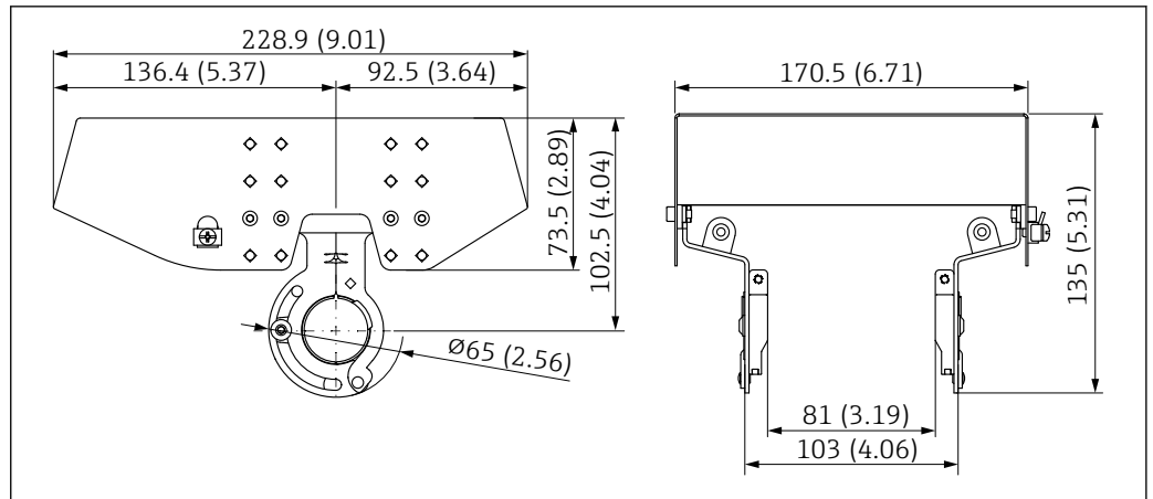
図 39 日除けカバー、SUS 316L 相当、XW112 の寸法。測定単位 mm (in)
