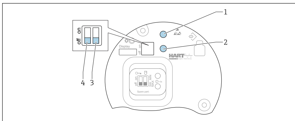
15 Betjeningstaster og DIP-kontakter på den elektroniske HART-indsats
