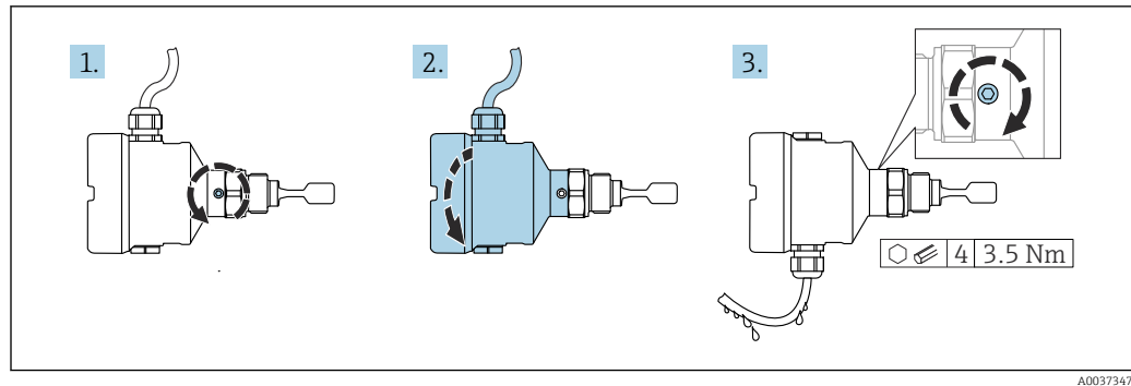
15 Caja con tornillo de bloqueo externo y circuito de goteo
