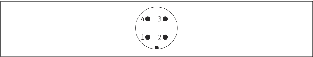
20 Conector M12, asignación de pines
