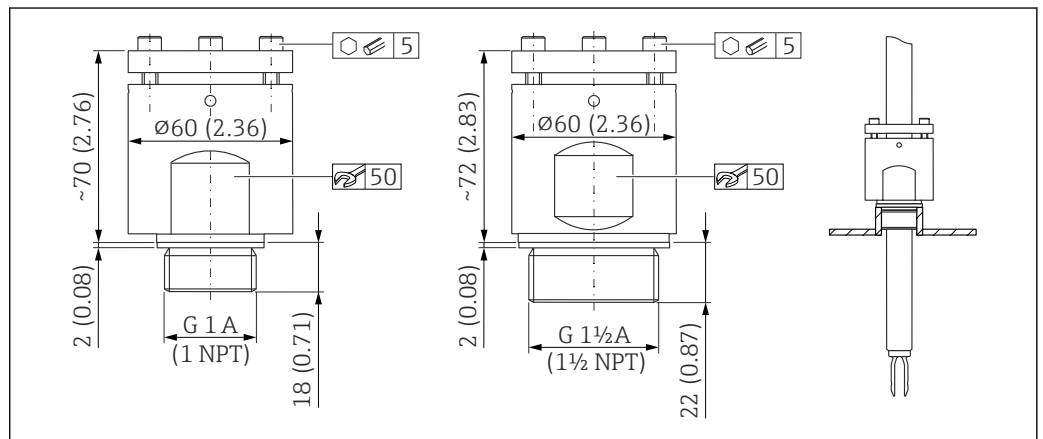
33 Casquillos deslizantes para alta presión. Unidad de medida mm (in)
