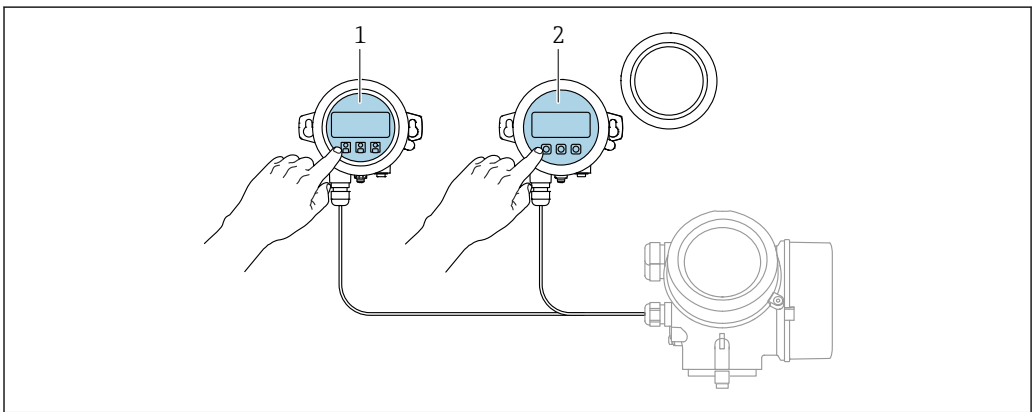
36 FHX50 的操作选项 1 显示与操作单元 SD03, 光敏键操作, 可以在玻璃盖板外部操作 2 显示与操作单元 SD02, 按键操作; 必须打开盖板
