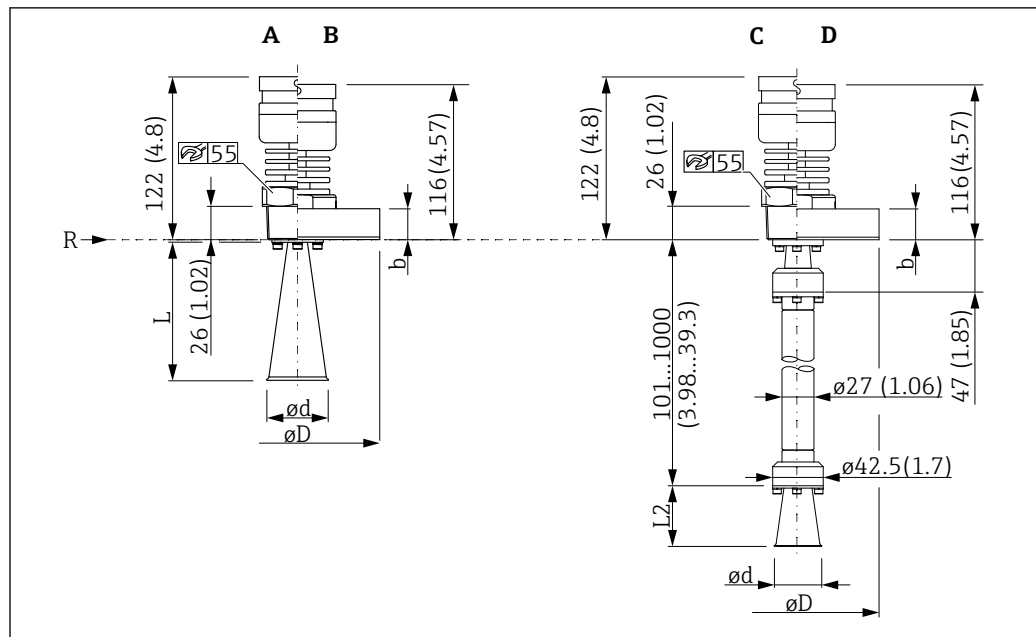
图 31 天线 ( T < 250\text{ °C} (482 °F)) 的外形尺寸示意图。测量单位 mm (in)
