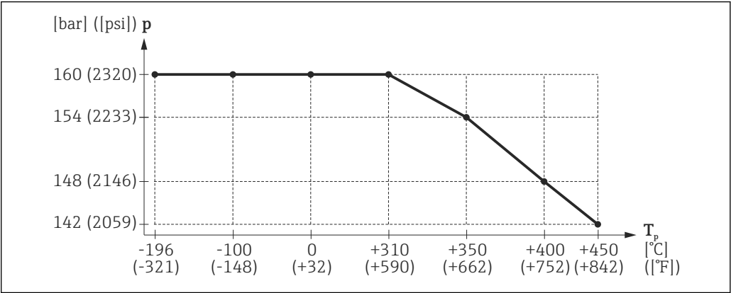
25 FMR51: 高温型仪表的允许过程温度和过程压力范围（订购选项 090 “密封圈”，选型代号 D2）
