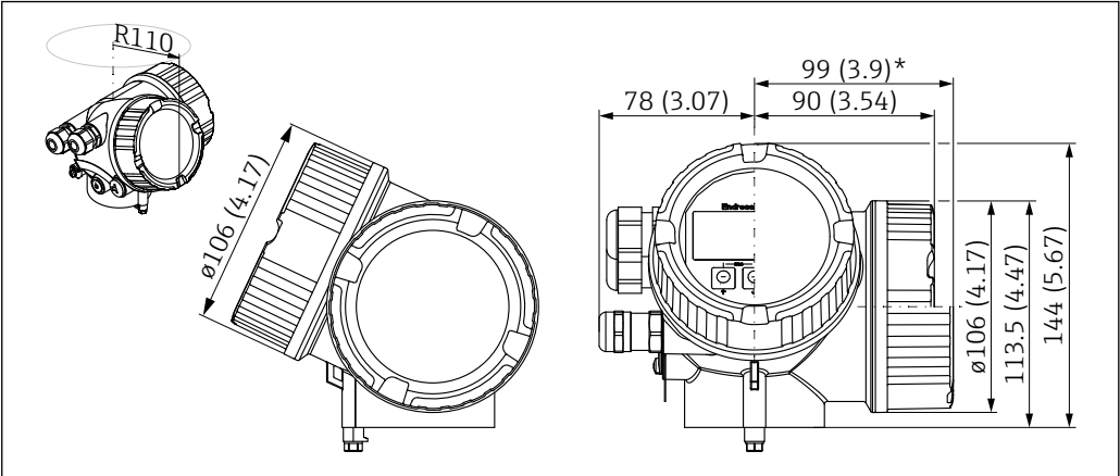
27 GT19 外壳 (塑料 PBT)。测量单位 mm (in)
