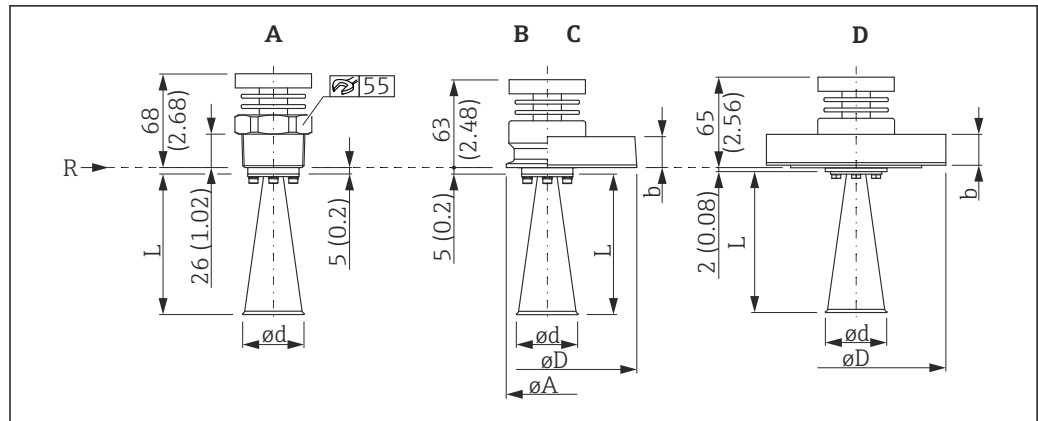
图 29 天线（无天线延伸管）的外形尺寸示意图。测量单位 mm (in)
