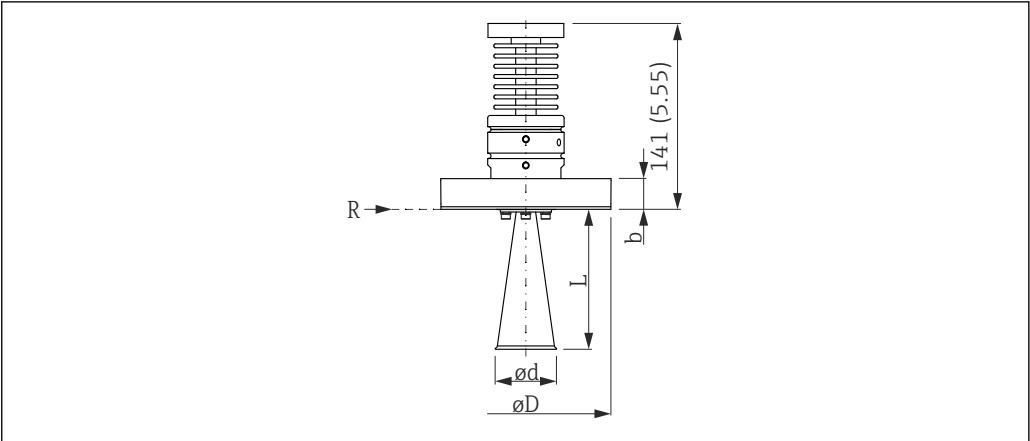
图 32 天线 ( T < 450\text{ }^{\circ}\text{C} (842 °F)) 的外形尺寸示意图。测量单位 mm (in)
