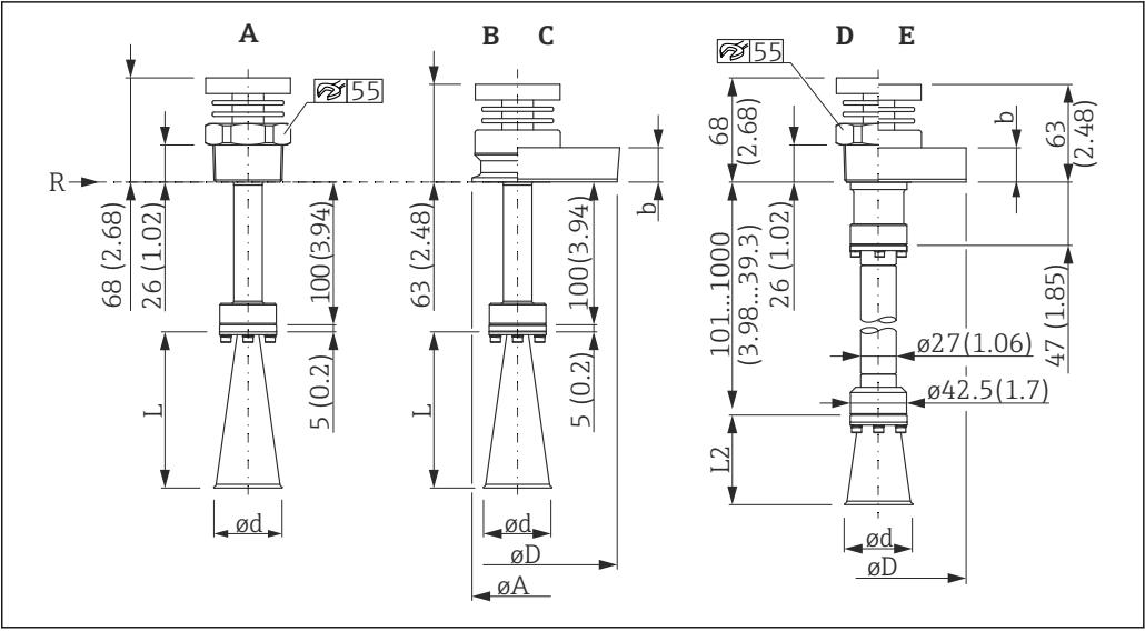
30 天线（带天线延伸管）的外形尺寸示意图。测量单位 mm (in)
