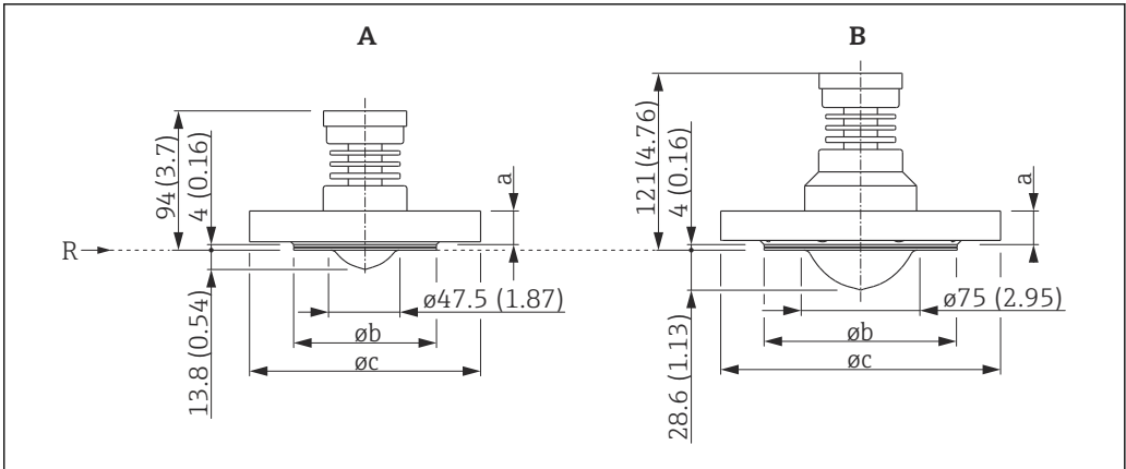
35 带法兰的仪表的外形尺寸示意图。测量单位 mm (in)
