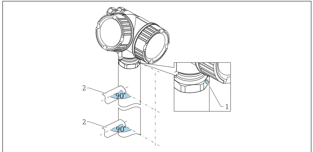
图 24 在旁通管中安装
