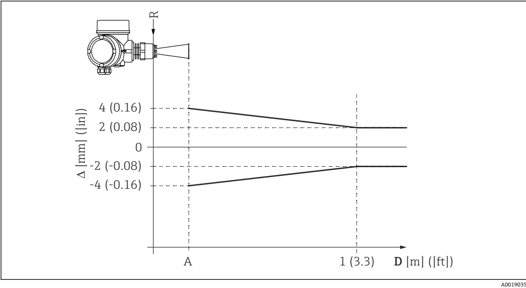
图 18 近距离测量时的最大测量误差; 图示为标准型仪表的参数值
