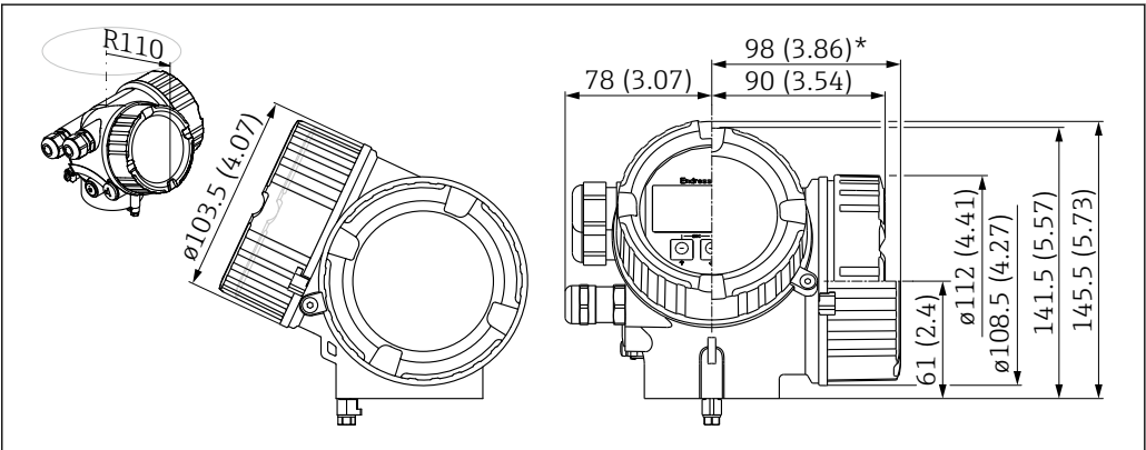
28 GT20 外壳 (铝, 带涂层)。测量单位 mm (in)
