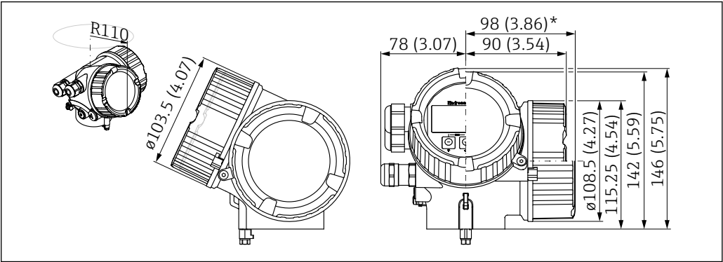
26 GT18 外壳 (316 L)。测量单位 mm (in)
