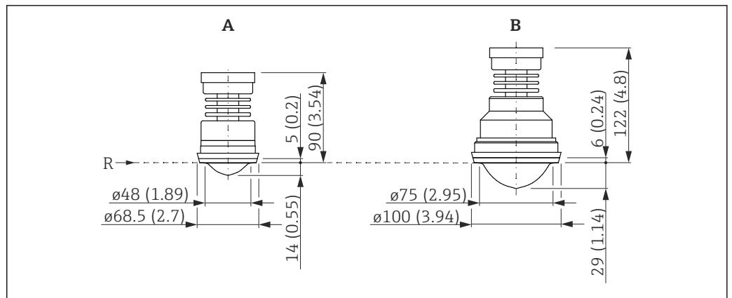
图 33 带 DIN11851 牛奶管道接头的仪表的外形尺寸示意图。测量单位 mm (in)
