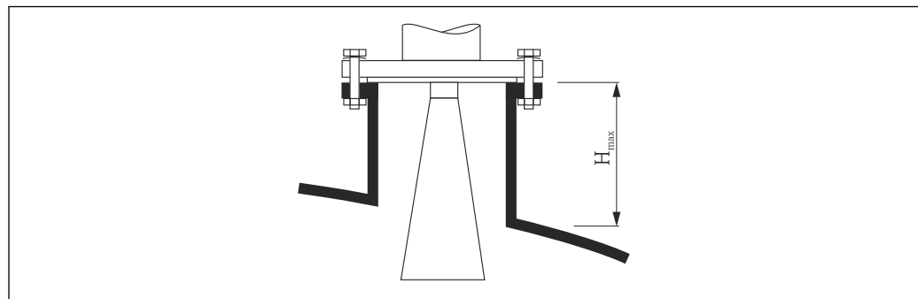
图 21 喇叭天线的安装短管高度（FMR51）示意图
