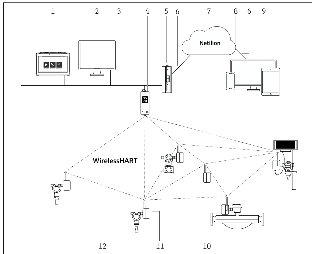
図 1 FieldGate SWG50 を使用した WirelessHART ネットワークの構成例
