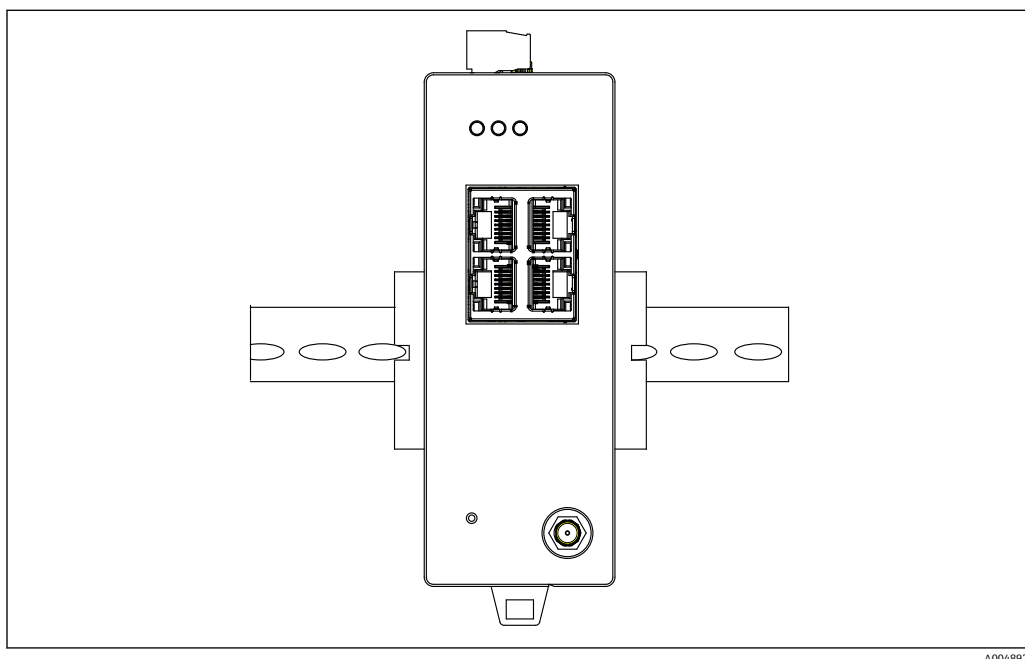
図 2 標準的な DIN レールへの取付け
