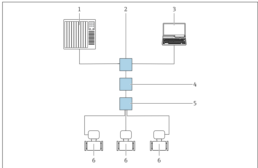
31 Options de configuration à distance via Modbus TCP sur protocole Ethernet-APL (active)
