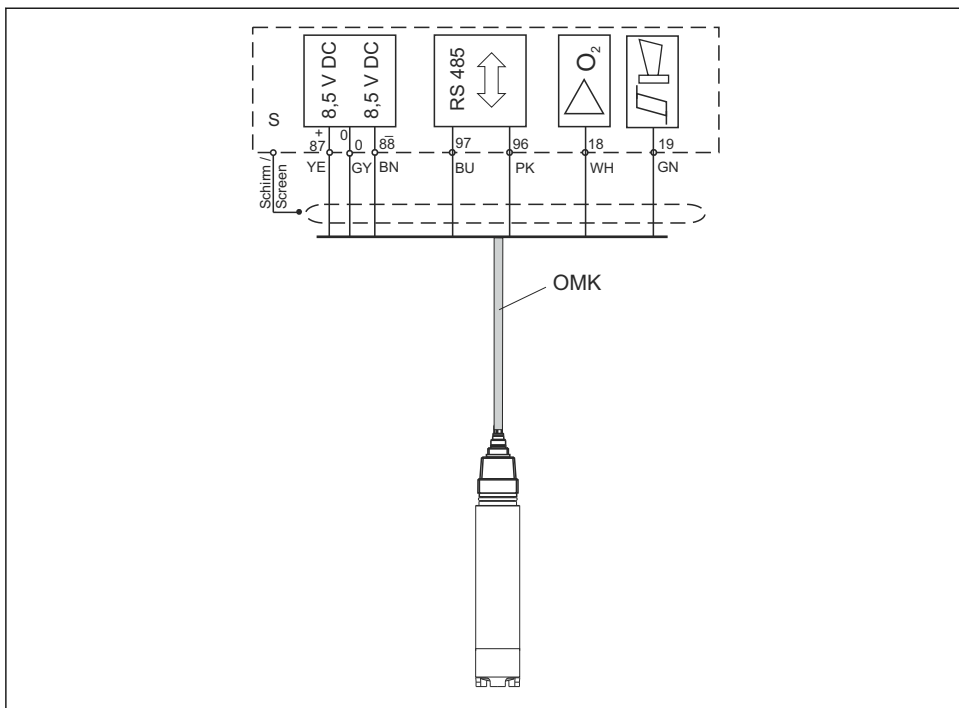
13 Anslutningsexempel: COS31/71 med OMK-kabel
