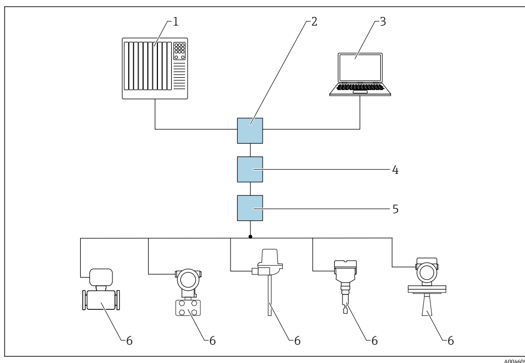
図 10 PROFINET over Ethernet-APL ネットワーク経由のリモート操作用オプション：スター型トポロジー
