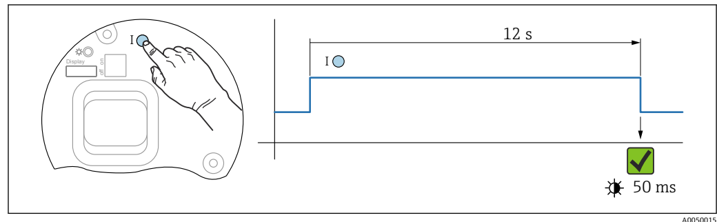
図 14 工場設定へのリセット手順
