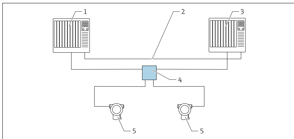
図 11 冗長システム (S2) のレイアウト例：スター型トポロジー
