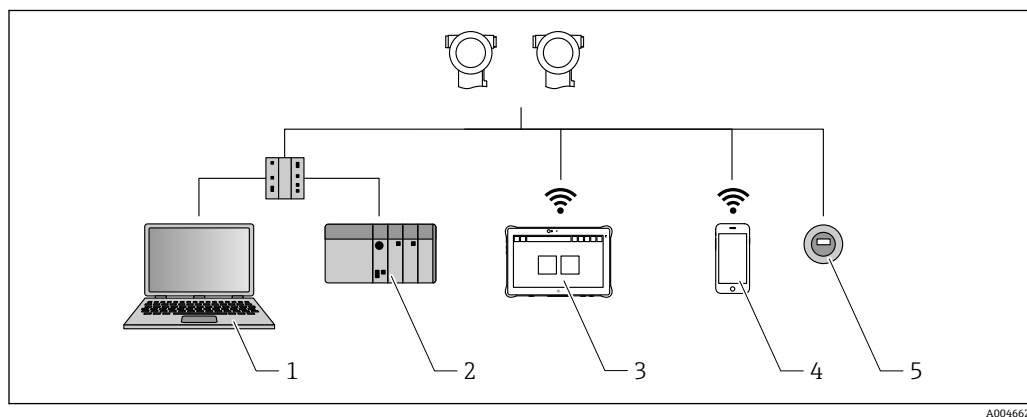
図 12 PROFINET プロトコル経由のリモート操作用オプション
