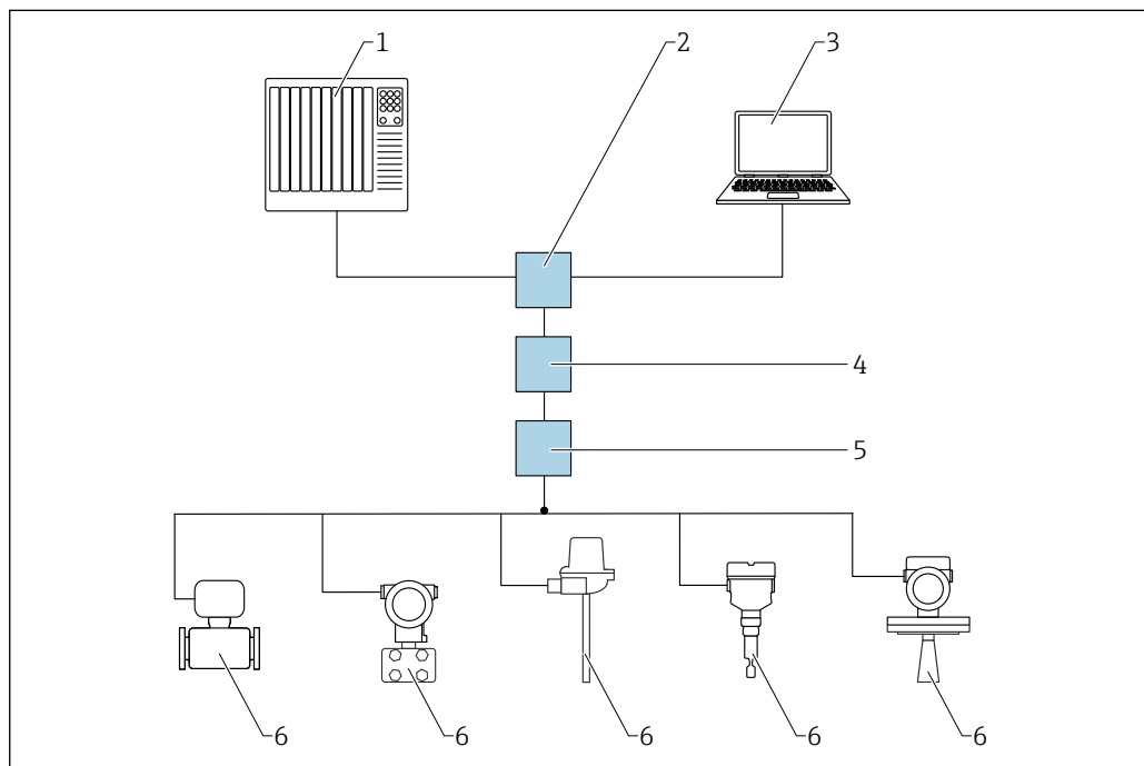
図 9 PROFINET over Ethernet-APL ネットワーク経路のリモート操作オプション: スター型トポロジー
