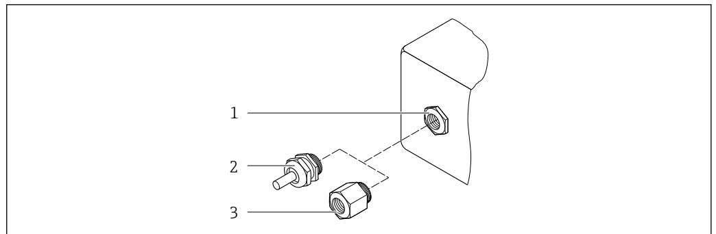
45 Возможные варианты кабельных вводов / кабельных уплотнений
