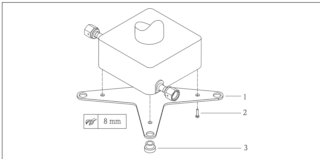
8 Монтажный комплект для монтажной пластины Cubemass
