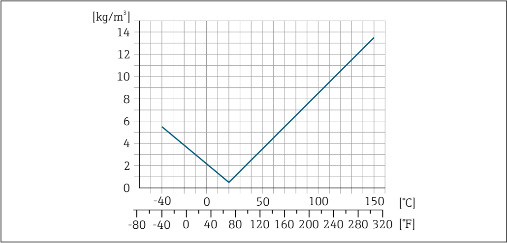
41 Калибровка по плотности на месте эксплуатации, в примере при +20 °C (+68 °F)
