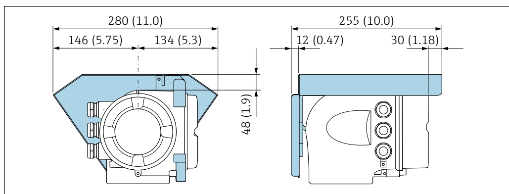
11 Защитный козырек от погодных явлений для Proline 500 – единица измерения- мм (дюймах)
