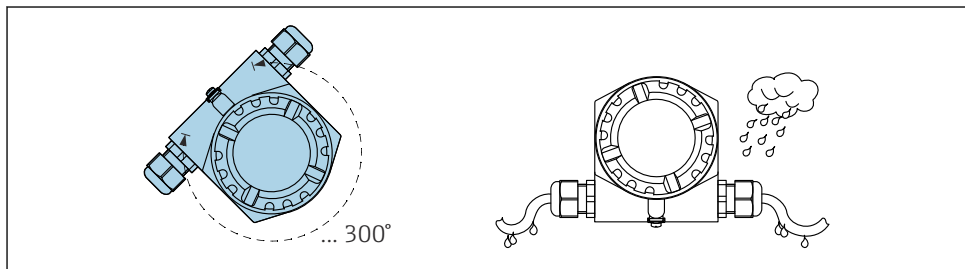
14 Gehäuse ohne Feststellschraube; Abtropfschlaufe am Kabel formen
