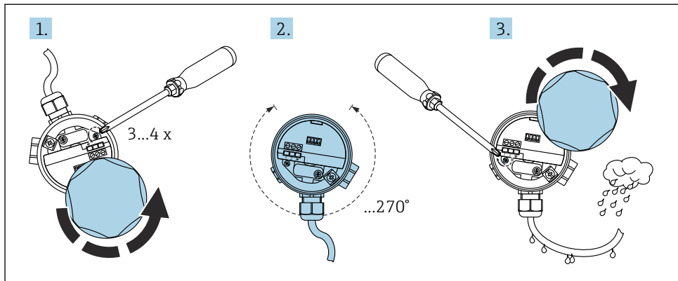
13 Gehäuse mit Feststellschraube; Abtropfschlaufe am Kabel formen
