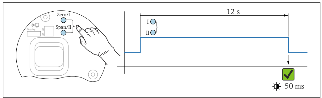
图 11 电子插件上的操作按键
