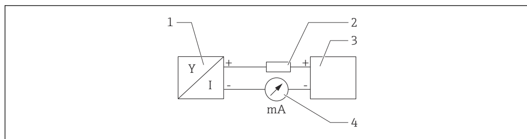
图 3 HART 接线框图
