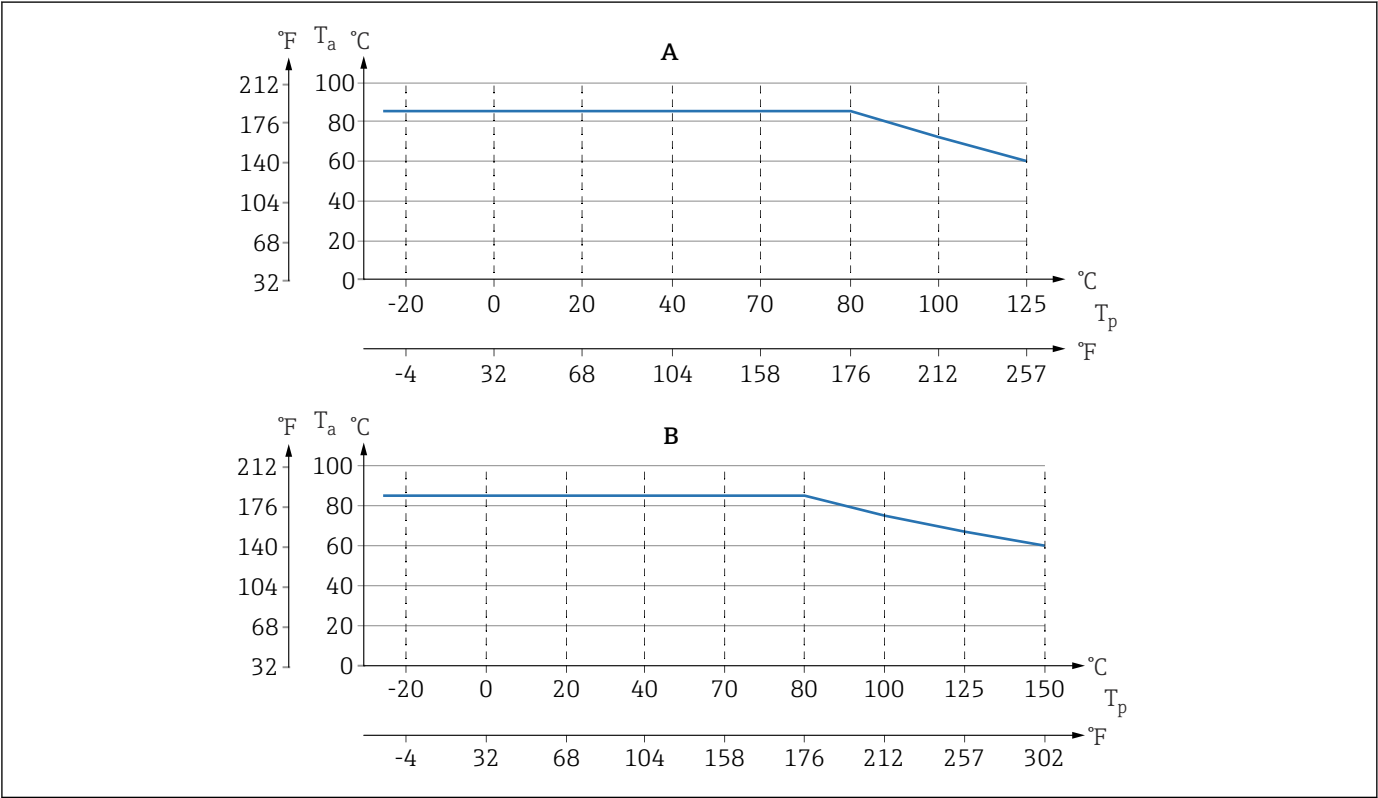
12 Les valeurs sont valables pour un montage vertical sans isolation. A Toutes les versions sauf B B "Version haute température" Tp Température de process Ta Température ambiante
