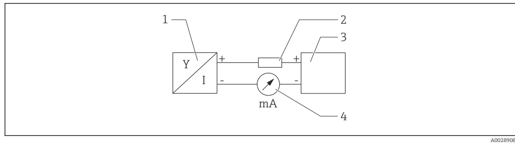
3 Schéma de principe du raccordement HART
