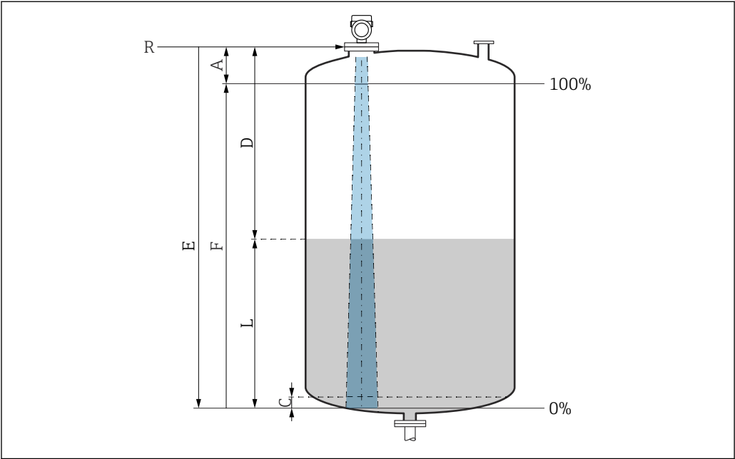
图 13 液位测量的设置参数
