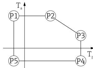
图 41 316L 外壳; 过程温度范围: -10 ... +200 °C (+14 ... +392 °F)
