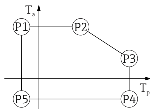
图 32 塑料外壳；过程温度范围：-40 ... +200 °C (-40 ... +392 °F)
