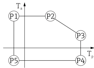
图 45 316L 外壳; 过程温度范围: -40 ... +200 °C (-40 ... +392 °F)
