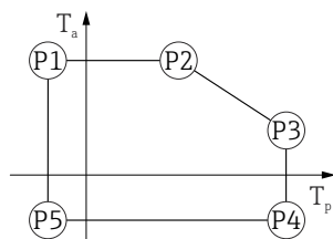
图 24 塑料外壳；过程温度范围：-10 ... +200 °C (+14 ... +392 °F)
