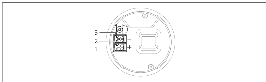
图 4 接线腔内的接线端子和接地端，单腔室外壳
