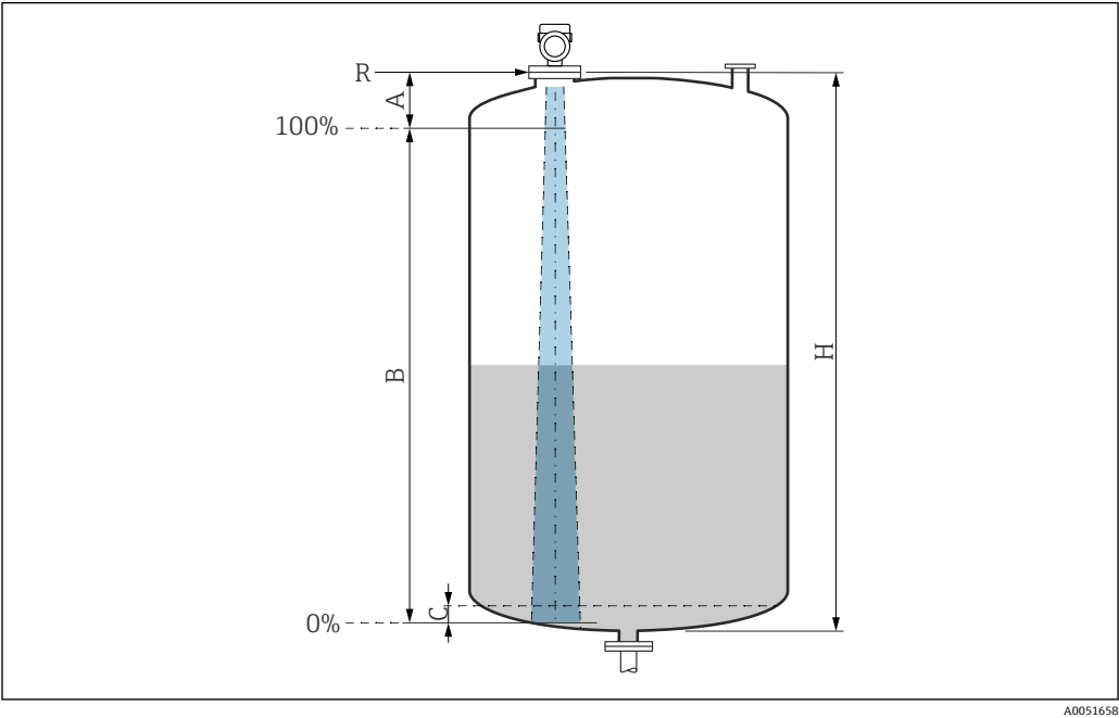
图 21 有效测量范围
