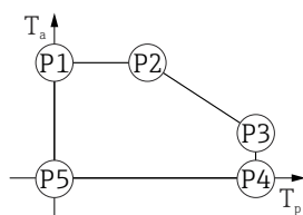
图 33 塑料外壳；过程温度范围：0 ... +200 °C (+32 ... +392 °F)，适用 CSA C/US 认证型仪表
