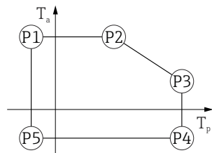
图 50 316L 外壳，卫生型；过程温度范围：-40 ... +150 °C (-40 ... +302 °F)
