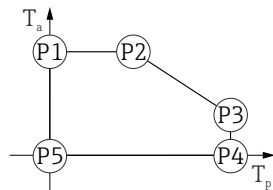
图 25 塑料外壳；过程温度范围：0 ... +200 °C (+32 ... +392 °F)，适用 CSA C/US 认证型仪表
