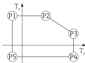
图 28 塑料外壳；过程温度范围：-20 ... +200 °C (-4 ... +392 °F)
