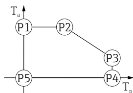
图 23 塑料外壳；过程温度范围：0 ... +150 °C (+32 ... +302 °F)，适用 CSA C/US 认证型仪表
