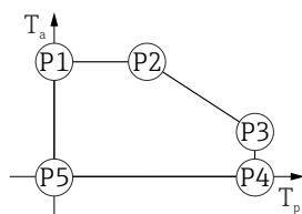
图 31 塑料外壳；过程温度范围：0 ... +150 °C (+32 ... +302 °F)，适用 CSA C/US 认证型仪表
