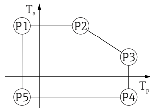
图 51 316L 外壳，卫生型；过程温度范围：-40 ... +200 °C (-40 ... +392 °F)
