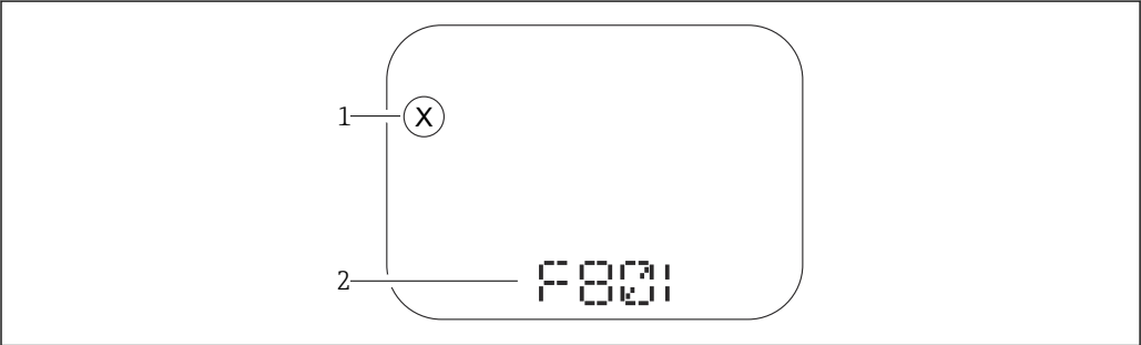
图 15 段码显示屏，无按键 1 状态图标（事件类别图标） 2 状态信号及诊断事件
