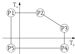
图 44 316L 外壳; 过程温度范围: -40 ... +150 °C (-40 ... +302 °F)
