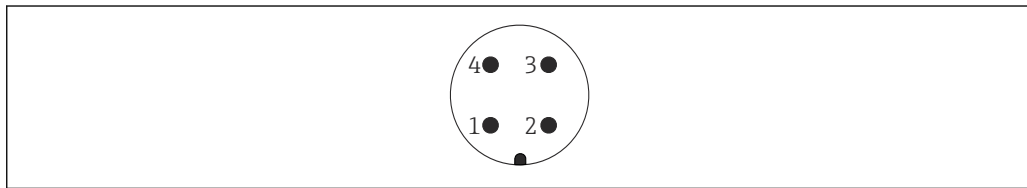
图 7 仪表连接插头示意图
