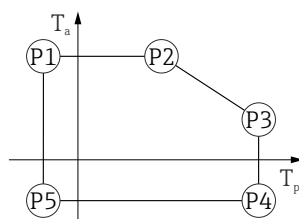
图 30 塑料外壳；过程温度范围：-40 ... +150 °C (-40 ... +302 °F)
