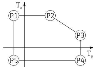
图 26 塑料外壳；过程温度范围：-20 ... +150 °C (-4 ... +302 °F)
