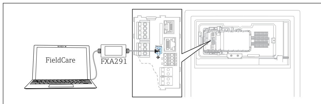
51 Anschlussübersicht
