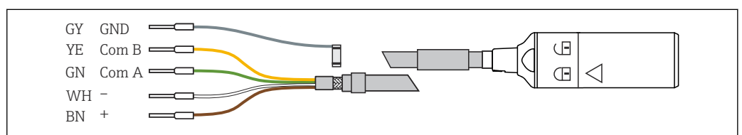
25 Beispiel Memosens-Datenkabel CYK10
