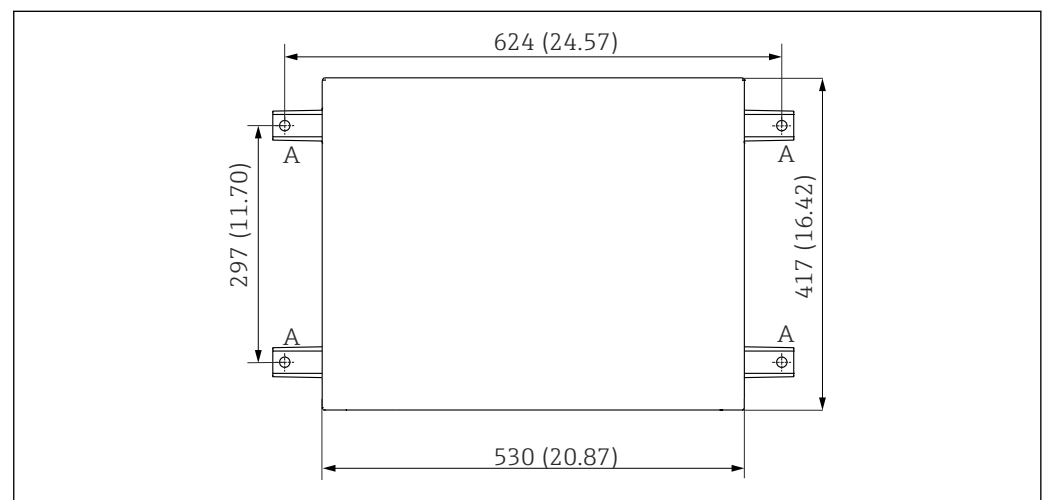
16 Fundamentplan. Maßeinheit mm (in)
