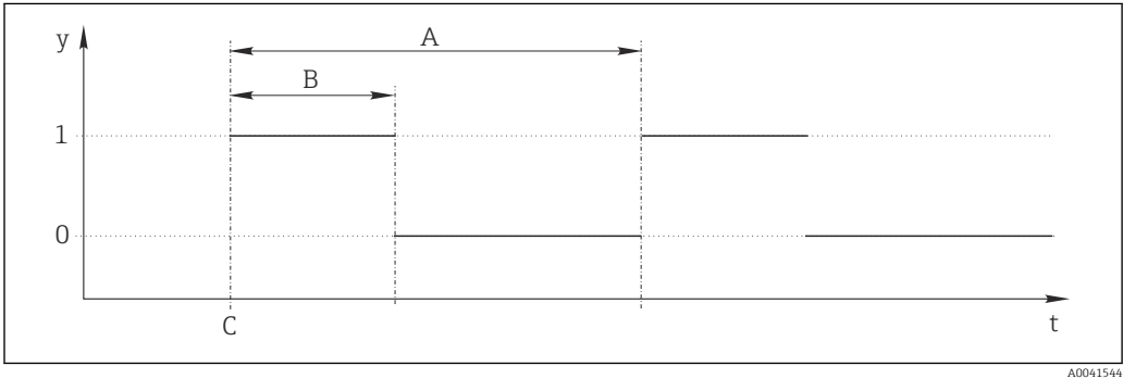
65 Signalverlauf eines Zeitgebers t Zeitachse y Signalpegel (1 = ein, 0 = aus) A Periode B Signaldauer C Startzeitpunkt (Startdatum, Startzeit)
