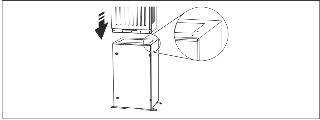
17 Befestigung Sockel
