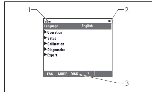
53 Display (Beispiel)
