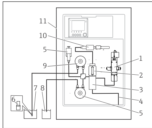
2 Messereinrichtung mit Liquiline System CA80TP und Saugkorb
