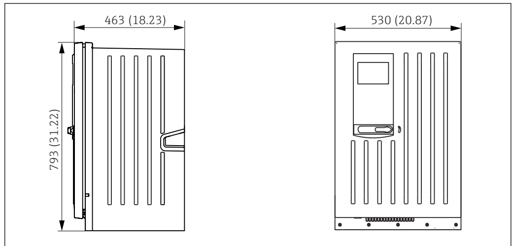
8 Geschlossener Aufbau. Maßeinheit mm (in)
