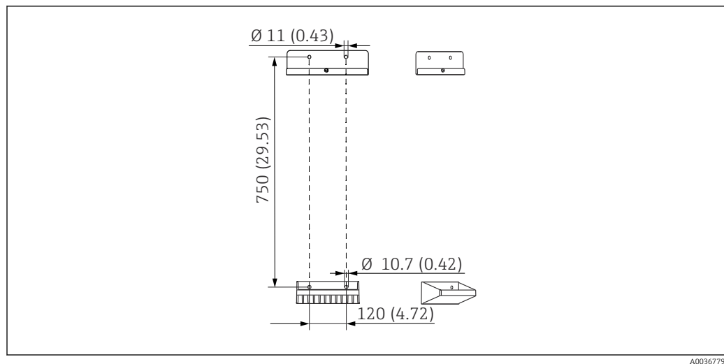
15 Abmessungen Halterung. Maßeinheit mm (in)
