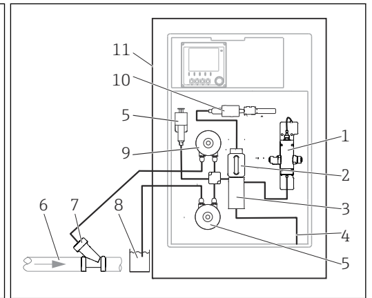
3 Messereinrichtung mit Liquiline System CA80TP und Y-Abscheider
