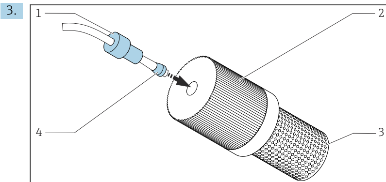
56 Mitgelieferten Saugkorb an Probenschlauch montieren
