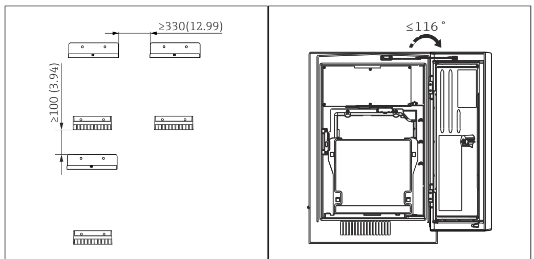
13 Notwendiger Montageabstand. Maßeinheit mm (in)
