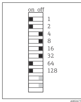
47 Gültige Modbus-Adresse 195
