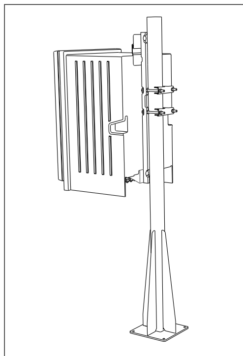
20 An Mast montierter Analysator (von hinten)
