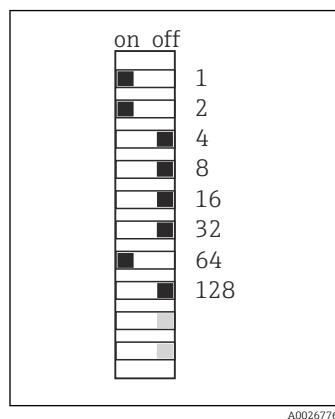
46 Gültige PROFIBUS-Adresse 67
