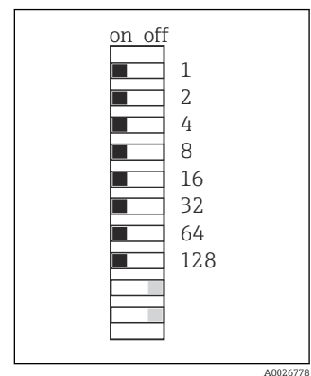
48 Ungültige Adresse 255 1)
