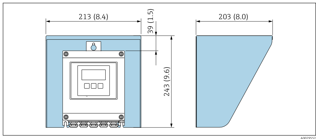
8 Capot de protection climatique pour Proline 500 – numérique ; unité mm (in)
