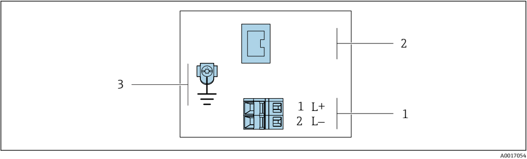
8 EtherNet/IP 型仪表的接线端子分配
