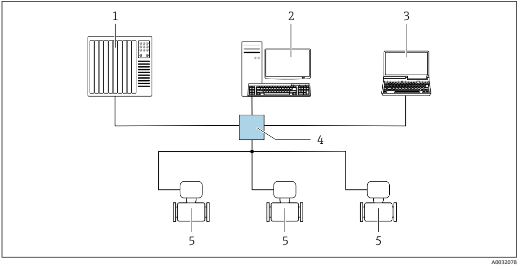
图 14 通过 EtherNet/IP 网络实现远程操作：星形拓扑结构
