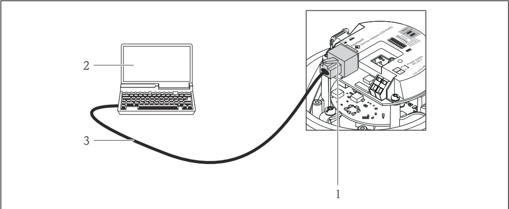
图 21 订购选项“输出”，选型代号 N: EtherNet/IP 1 测量设备的服务接口 (CDI -RJ45) 和 EtherNet/IP 接口，内置网页服务器访问接口 2 计算机，带网页浏览器 (例如 Internet Explorer)，用于访问设备内置网页服务器或“FieldCare”、“DeviceCare”调试软件，带 COM DTM “CDI 通信 TCP/IP” 3 标准以太网连接电缆，带 RJ45 插头
