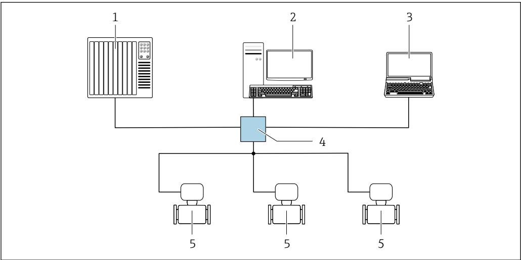
图 20 通过 EtherNet/IP 网络实现远程操作：星形拓扑结构
