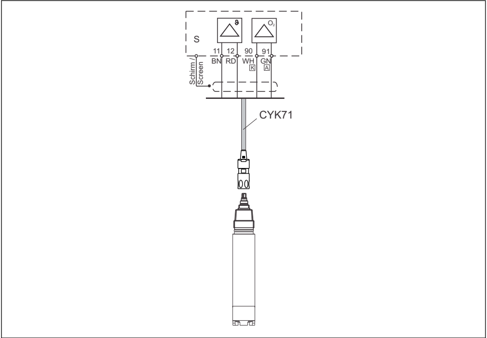
9 Bağlantı örneği: COS41 ile CYK71 kablosu
