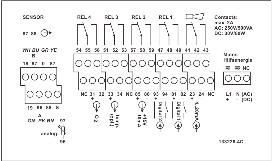
11 Liquisys M bağlantı bölgesi etiketi, WX/WS versiyonu
