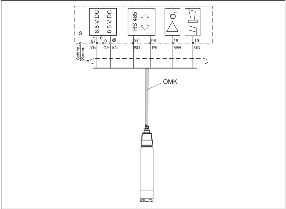
13 Bağlantı örneği: OMK kablosu ile COS31/71
