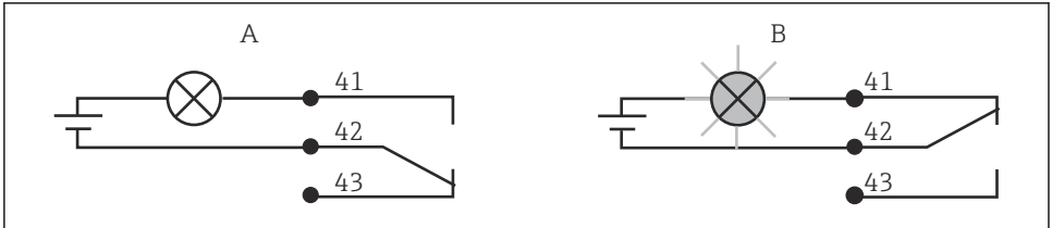
14 Tavsiye edilen arıza emniyetli alarm bağlantı anahtarı
