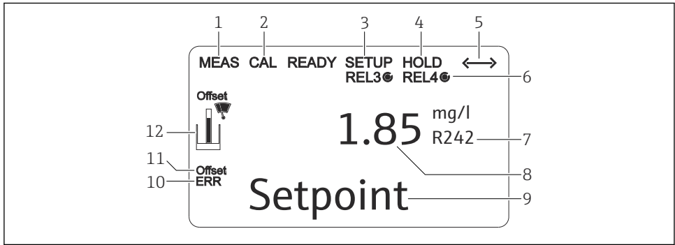
15 Transmitter LC ekranı
