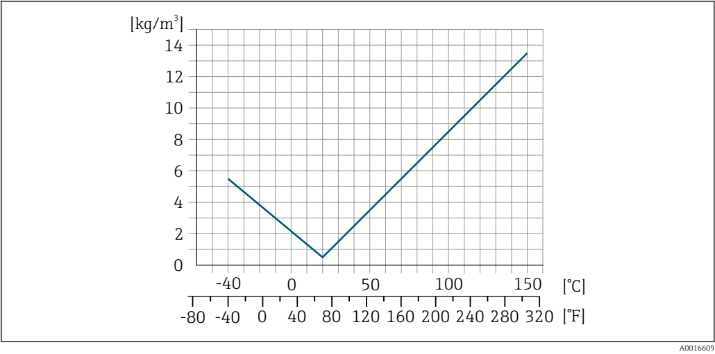
34 Ajustage sur site de la masse volumique, par exemple à +20 °C (+68 °F)
