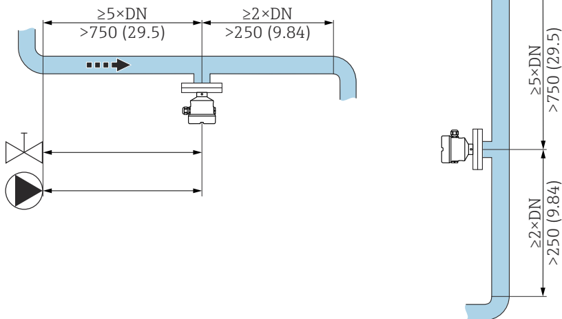
8 Installera inloppssträckan. Mått enhet mm (in)
