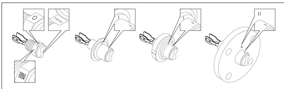
13 Stängaffelns läge vid horisontell installation i kärlet med hjälp av markeringen
