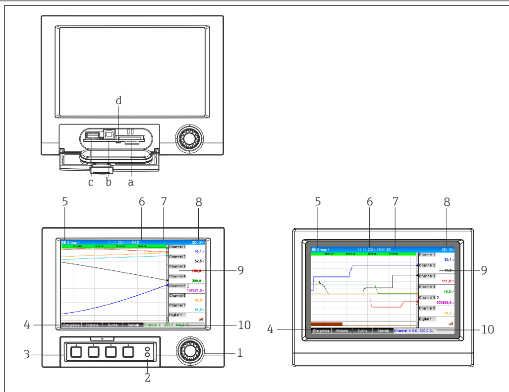
19 Face avant de l'appareil (gauche : version avec navigateur et interfaces en face avant ; droite : version avec face avant en inox et commande tactile)
