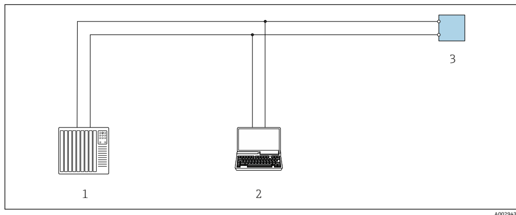
図 31 Modbus RS485 プロトコル経由のリモート操作用オプション（アクティブ）
