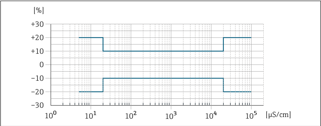
39 測定誤差 (標準)
