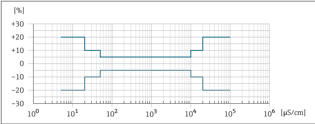
図 40 測定誤差（オプション：「校正済導電率測定」のオーダーコード、オプション CW）
