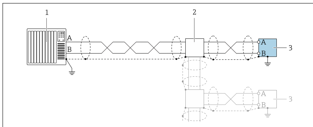
図 24 Modbus RS485 の接続例
