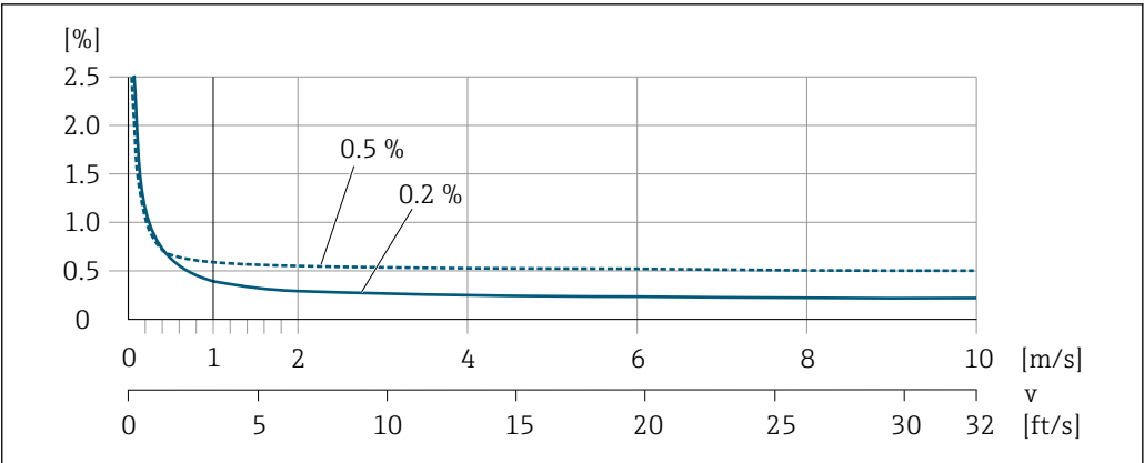
38 最大測定誤差 (% o.r.)
