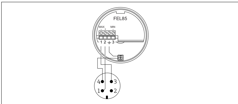
14 Klemmeplassering med M12-kontakt, MAX-driftsmodus
