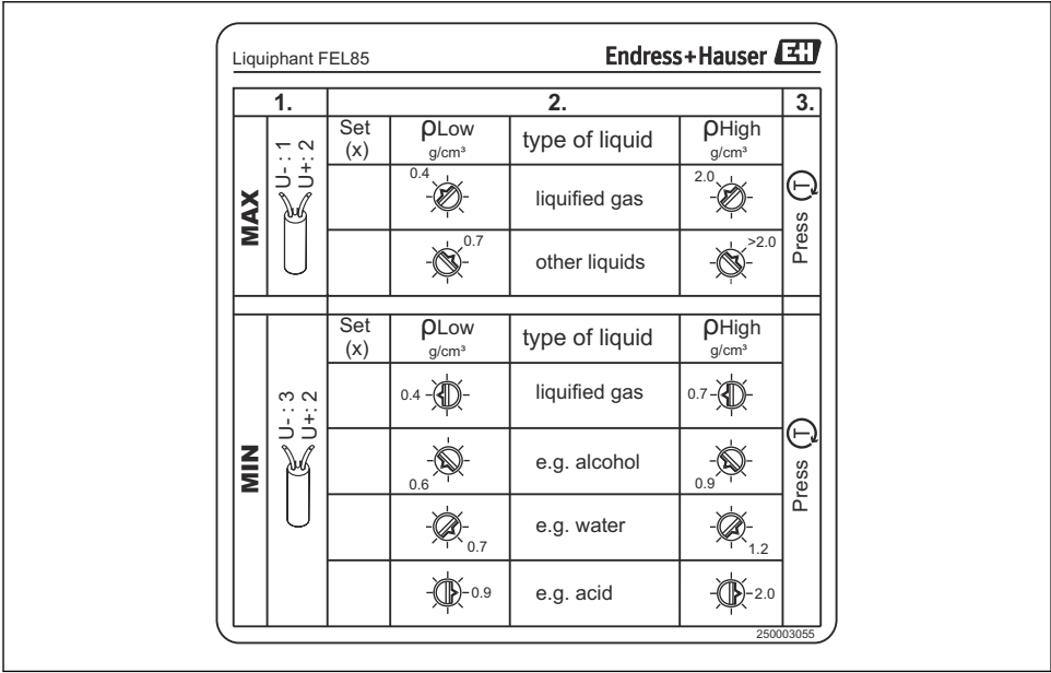
Figur: sensorkort
