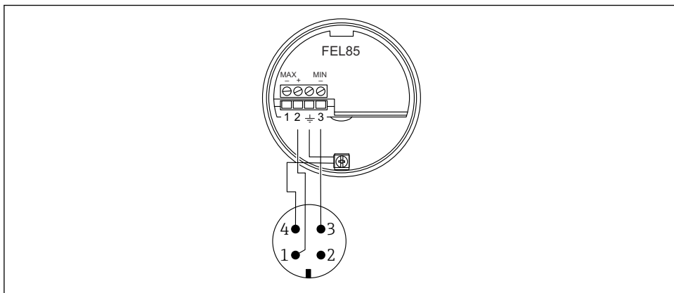
15 Klemmetilordning med M12-kontakt, MIN-driftsmodus
