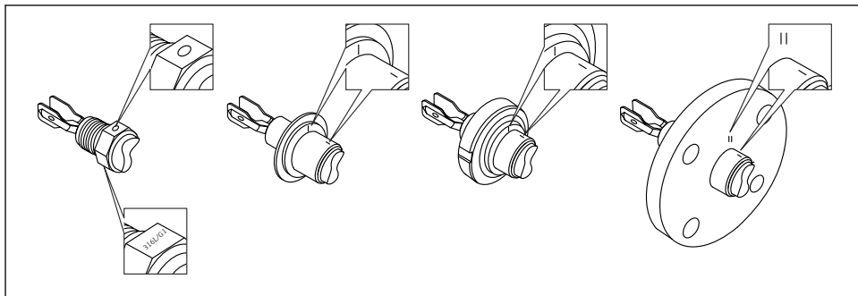
10 Stemmegaffelens posisjon når den installeres horisontalt i beholderen med merkingen
