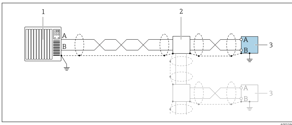
27 Пример подключения для Modbus RS485
