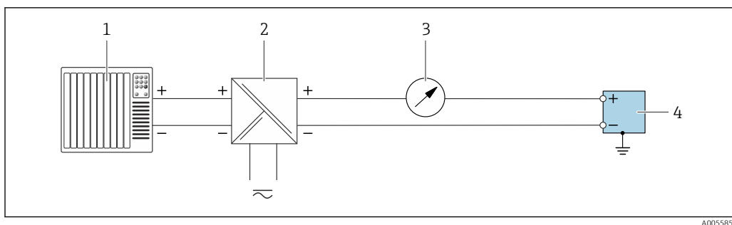
21 Пример подключения для токового выхода 4 до 20 мА (пассивного)
