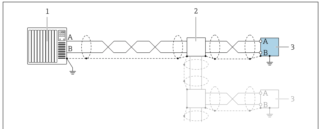
27 Ejemplo de conexión para Modbus RS485
