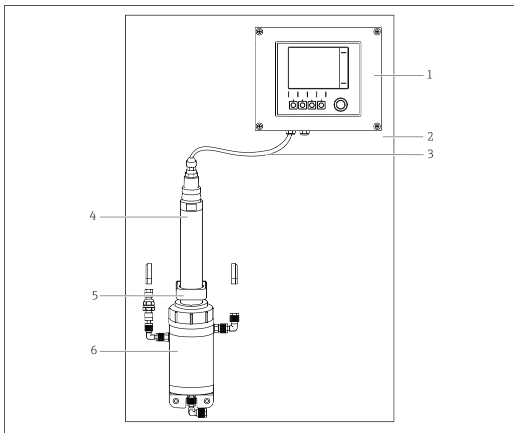
13 Ensemble de mesure
