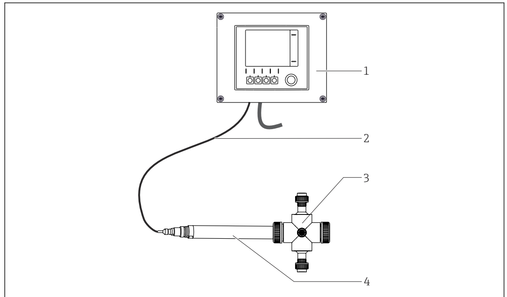
12 Exemple d'ensemble de mesure
