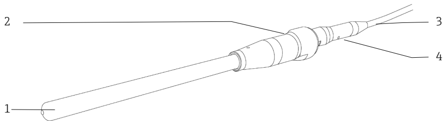
Figura 1. Configurazione non flangiata con cavo con canale in fibre
