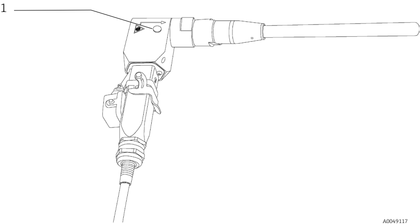
Figura 2. Indicatore laser a LED (1) sul gruppo del connettore in fibra ad angolo retto EO
