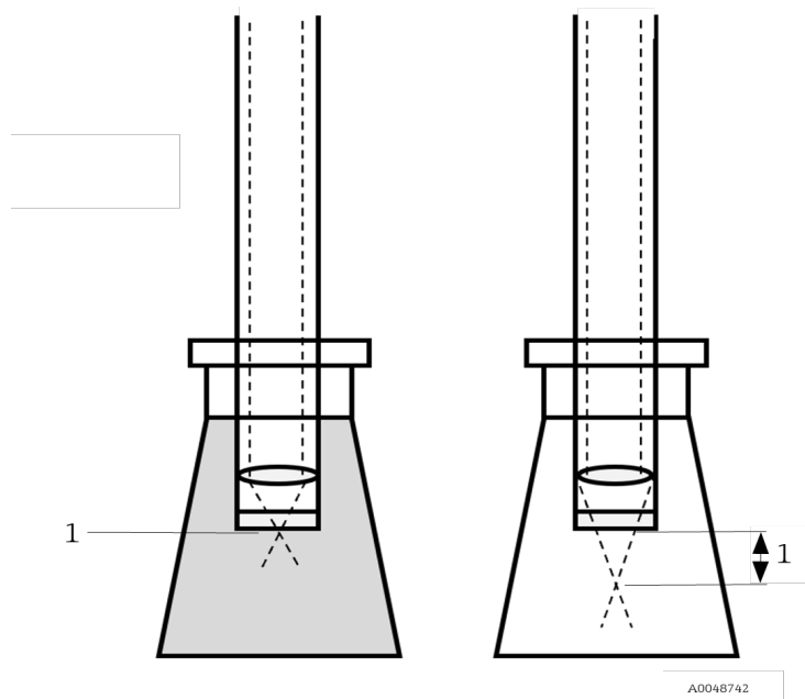
Figura 5. Confronto tra zona di raccolta dati corta (a sinistra) e lunga (a destra) (1)
