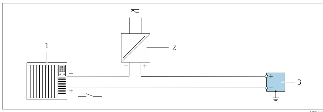
25 Пример подключения для входного сигнала состояния
