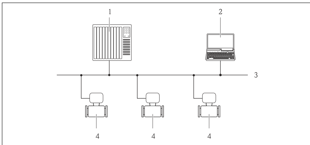
31 Варианты дистанционного управления через сеть PROFIBUS DP
