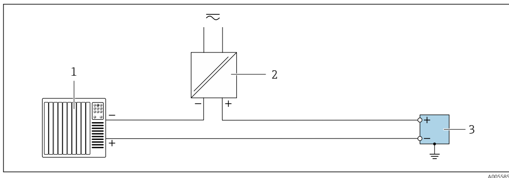
24 Пример подключения для релейного выхода
